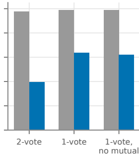
FiQA
