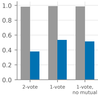
SciDocs
