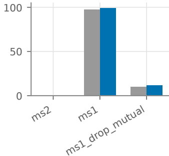
SciDocs
