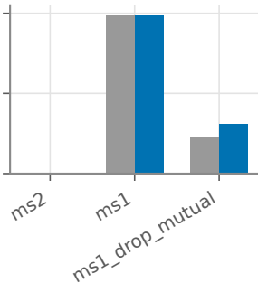
FiQA
