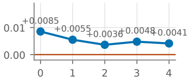
(B) SciDocs
