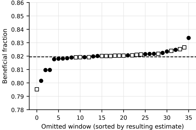
(d) Leave-one-window-out: beneficial fraction
