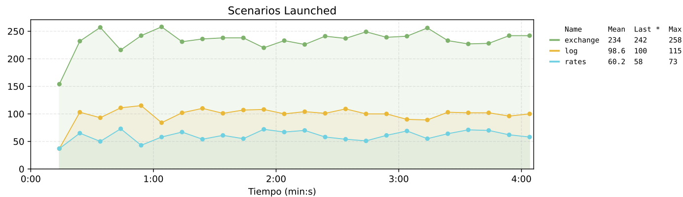
Figura 10. Escenarios del sistema base.
