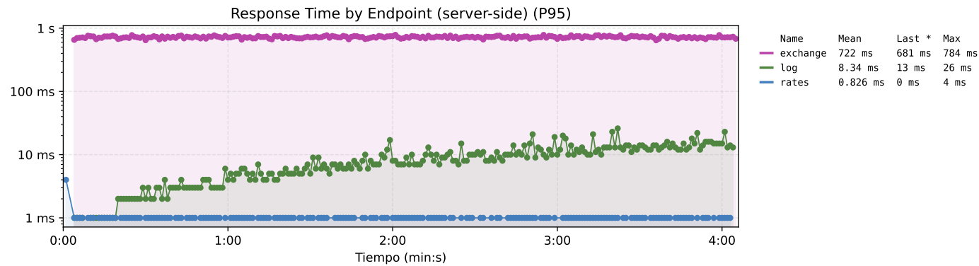
Figura 11. Tiempo de respuesta por endpoint del sistema base.
