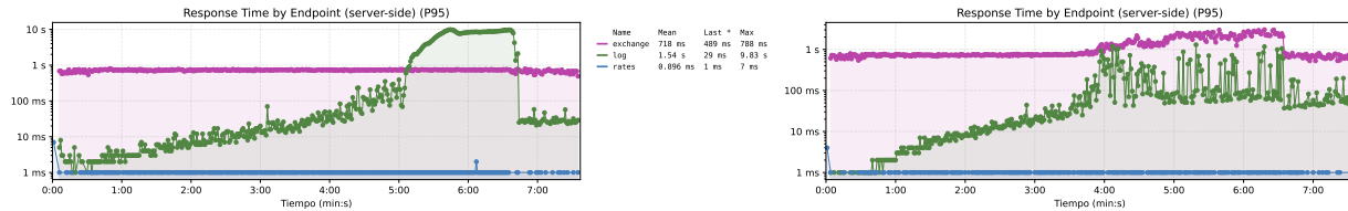
Figura 5. Comparativa de los resultados de latencia por endpoint entre la propuesta 1 (izquierda) y el sistema base (derecha) frente a un escenario de stress. Con diferencia el analisis mas interesante, la propuesta 1 permitio como se esperaba mejorar la latencia en el endpoint de exchange, se puede notar que este no se ve afectado por la degradacion del endpoint de logs. Como si ocurría en el caso base, donde al rededor del minuto 4, los tiempos de respuesta de exchange incrementaban, en este caso, los tiempos de respuesta se mantienen estables en 1 segundo, acotado por la dependencia del servicio externo. Por otro lado, los tiempos de respuesta de /log empeoraron, sinembargo es esperable, la mayor disponibilidad antes mencionada implica que se registraron mas transacciones, por lo que el tamaño del log necesariamente aumento. Esto explica el aumento de los tiempos de respuesta visto desde el lado del cliente antes mencionados, sinembargo, las metricas se ven ensuciadas al mezclar todos los endpoints.
