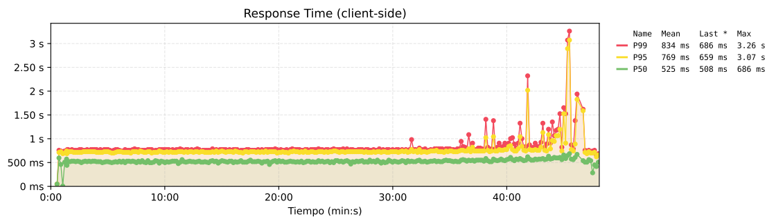
Figura 54. Tiempo de respuesta de la propuesta 1.
