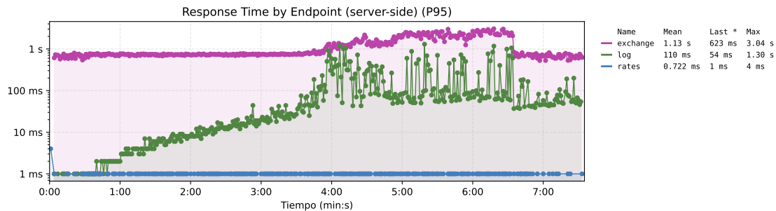
Figura 25. Tiempo de respuesta por endpoint del sistema base. El eje tiene una escala logarítmica.
