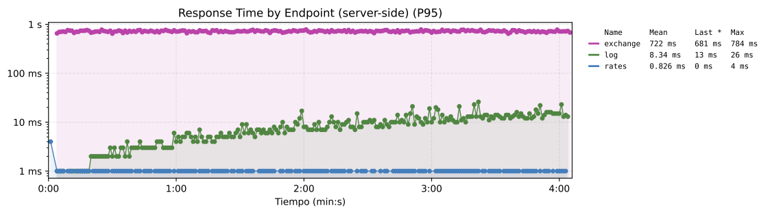
Figura 18. Tiempo de respuesta por endpoint del sistema base. El eje tiene una escala logaritmica.
