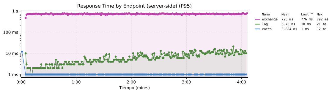
Figura 39. Tiempo de respuesta por endpoint de la propuesta 1. El eje tiene una escala logarítmica.
