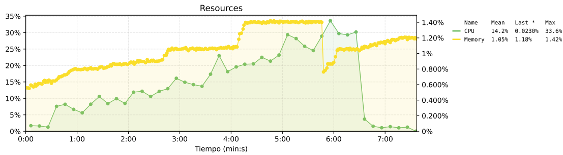
Figura 48. Estado de los recursos del nodo de exchange de la propuesta 1. El eje izquierdo muestra el uso de CPU, el eje derecho muestra el uso de memoria.
