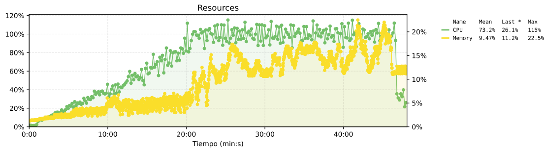
Figura 33. Estado de los recursos del sistema base. El eje izquierdo muestra el uso de CPU, el eje derecho muestra el uso de memoria.
