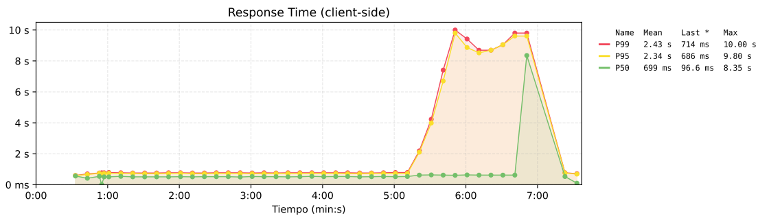
Figura 46. Tiempo de respuesta de la propuesta 1.
