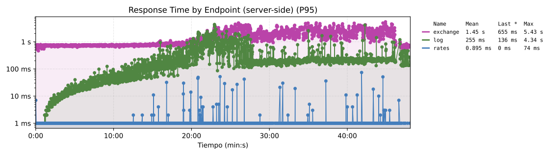
Figura 32. Tiempo de respuesta por endpoint del sistema base. El eje tiene una escala logarítmica.
