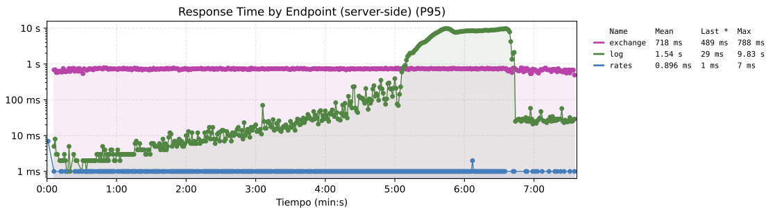
Figura 47. Tiempo de respuesta por endpoint de la propuesta 1. El eje tiene una escala logarítmica.
