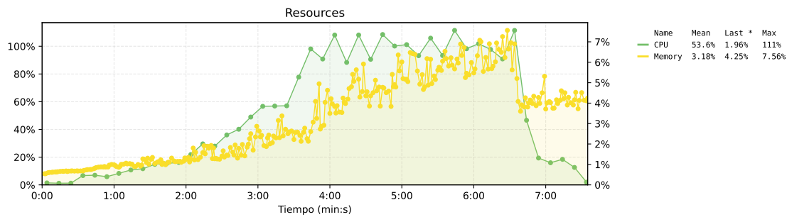
Figura 26. Estado de los recursos del sistema base. El eje izquierdo muestra el uso de CPU, el eje derecho muestra el uso de memoria.
