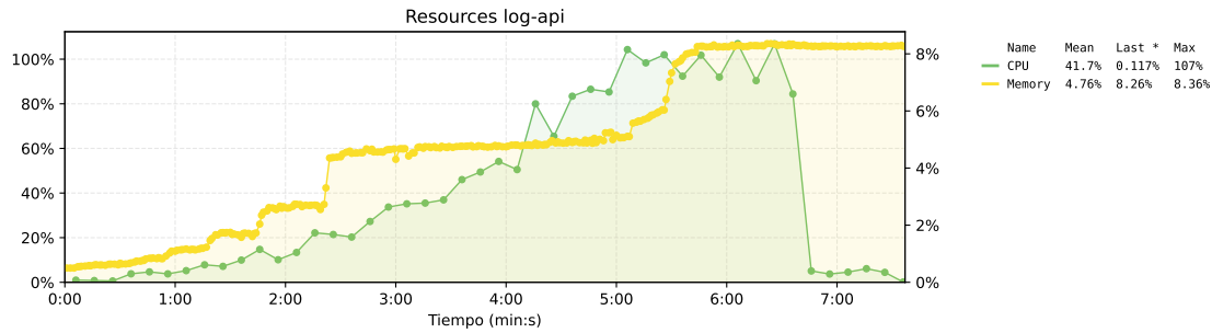
Figura 49. Estado de los recursos del nodo de logs de la propuesta 1. El eje izquierdo muestra el uso de CPU, el eje derecho muestra el uso de memoria.
