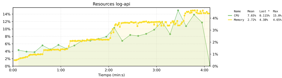
Figura 41. Estado de los recursos del nodo de logs de la propuesta 1. El eje izquierdo muestra el uso de CPU, el eje derecho muestra el uso de memoria.
