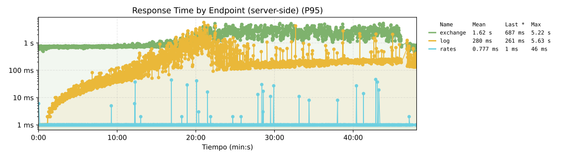
Figura 221. Tiempo de respuesta por endpoint de la propuesta 3. El eje tiene una escala logarítmica.
