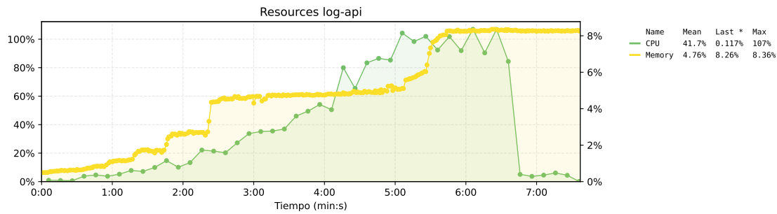
Figura 155. Estado de los recursos del nodo de logs de la propuesta 1. El eje izquierdo muestra el uso de CPU, el eje derecho muestra el uso de memoria.
