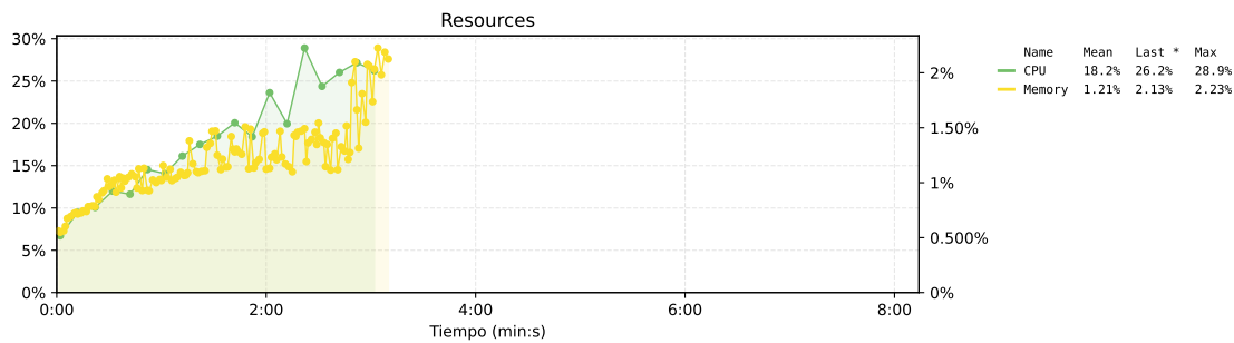
Figura 118. Estado de los recursos del sistema base. El eje izquierdo muestra el uso de CPU, el eje derecho muestra el uso de memoria.
