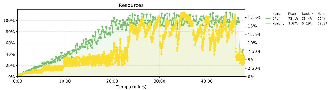
Figura 191. Estado de los recursos de la propuesta 2. El eje izquierdo muestra el uso de CPU, el eje derecho muestra el uso de memoria.
