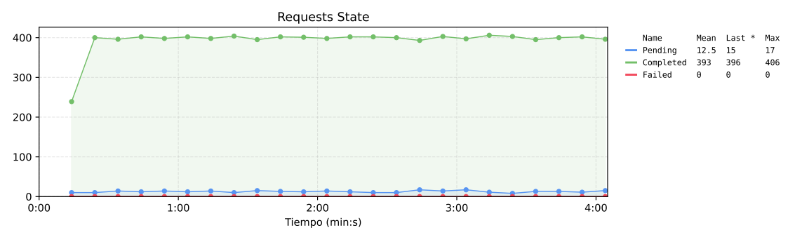
Figura 88. Estado de las requests del sistema base.
