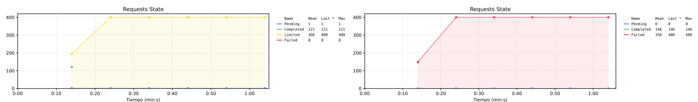
Figura 80. Comparativa de la disponibilidad ofrecida por la propuesta 3 (izquierda) y el sistema base (derecha) frente al escenario de concurrencia. Notar que el panel clasifica las respuestas 4xx como Limited : en la propuesta 3 los cambios sin fondos se informan como 409, mientras que en el sistema base se informaban como 500 ( Failed ). Como nuestra hipótesis indicaba el número de operaciones en el sistema base supera las 121 operaciones de cambio esperadas. Mientras que en la propuesta 3 acota perfectamente el número de operaciones completadas.
