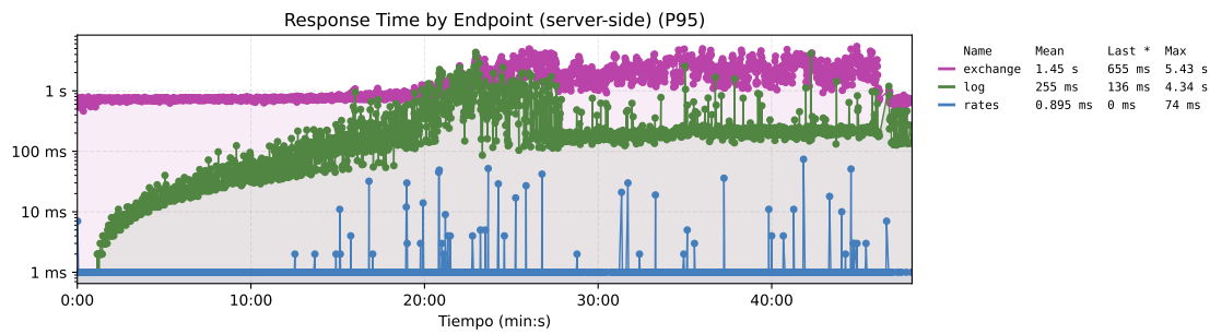
Figura 110. Tiempo de respuesta por endpoint del sistema base. El eje tiene una escala logarítmica.
