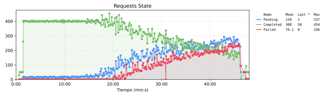
Figura 217. Estado de las requests de la propuesta 3.
