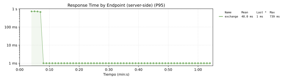
Figura 249. Tiempo de respuesta por endpoint de la propuesta 3. El eje tiene una escala logarítmica.
