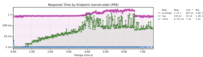
Figura 14. Se observa cómo el crecimiento en los tiempos de respuesta de /log, dado por el crecimiento del log, impacta directamente en la latencia del endpoint /exchange.
