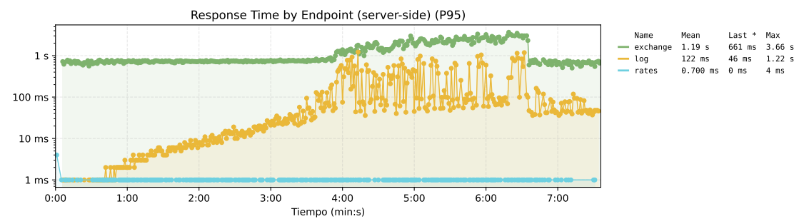
Figura 207. Tiempo de respuesta por endpoint de la propuesta 3. El eje tiene una escala logarítmica.
