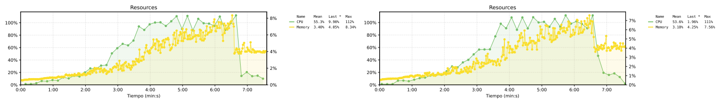
Figura 70. Comparativa de los resultados del uso de recursos entre la propuesta 3 (izquierda) y el sistema base (derecha) frente a un escenario de estrés. Se observan promedios de uso de CPU y de memoria muy similares. La propuesta mantiene el costo de uso de recursos.
