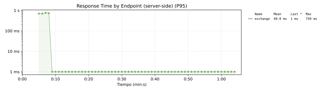
Figura 127. Tiempo de respuesta por endpoint del sistema base. El eje tiene una escala logarítmica.
