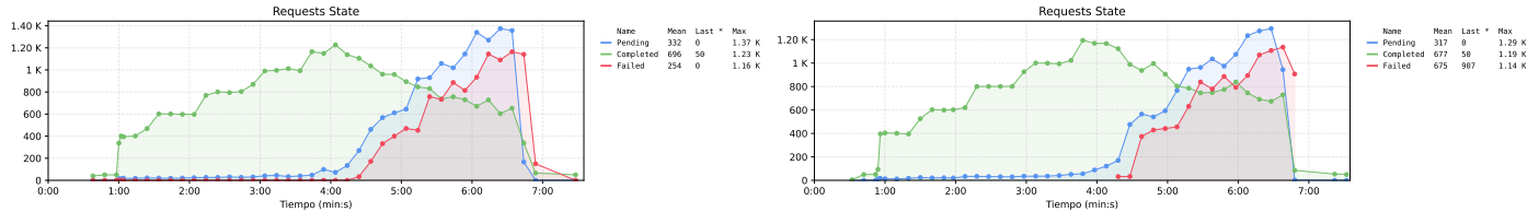
Figura 48. Comparativa de la disponibilidad ofrecida por la propuesta 2 (izquierda) y el sistema base (derecha) frente a un escenario de estrés. Ambos sistemas alcanzan su punto de quiebre en el mismo momento, alrededor del minuto 4:30, y presentan picos de fallas similares (1.16K frente a 1.14K por ventana). El promedio de respuestas satisfactorias por ventana es prácticamente el mismo (696 frente a 677). Como se esperaba, la táctica no mejora la disponibilidad frente a la sobrecarga.
