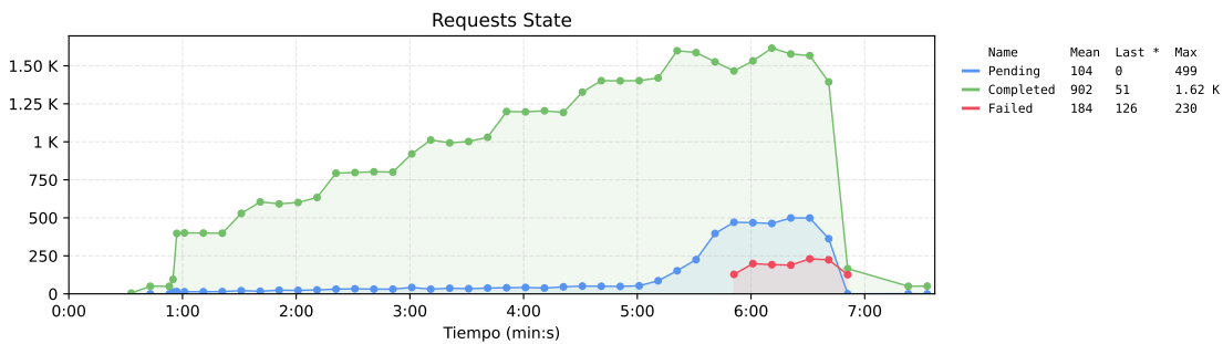
Figura 151. Estado de las requests de la propuesta 1.
