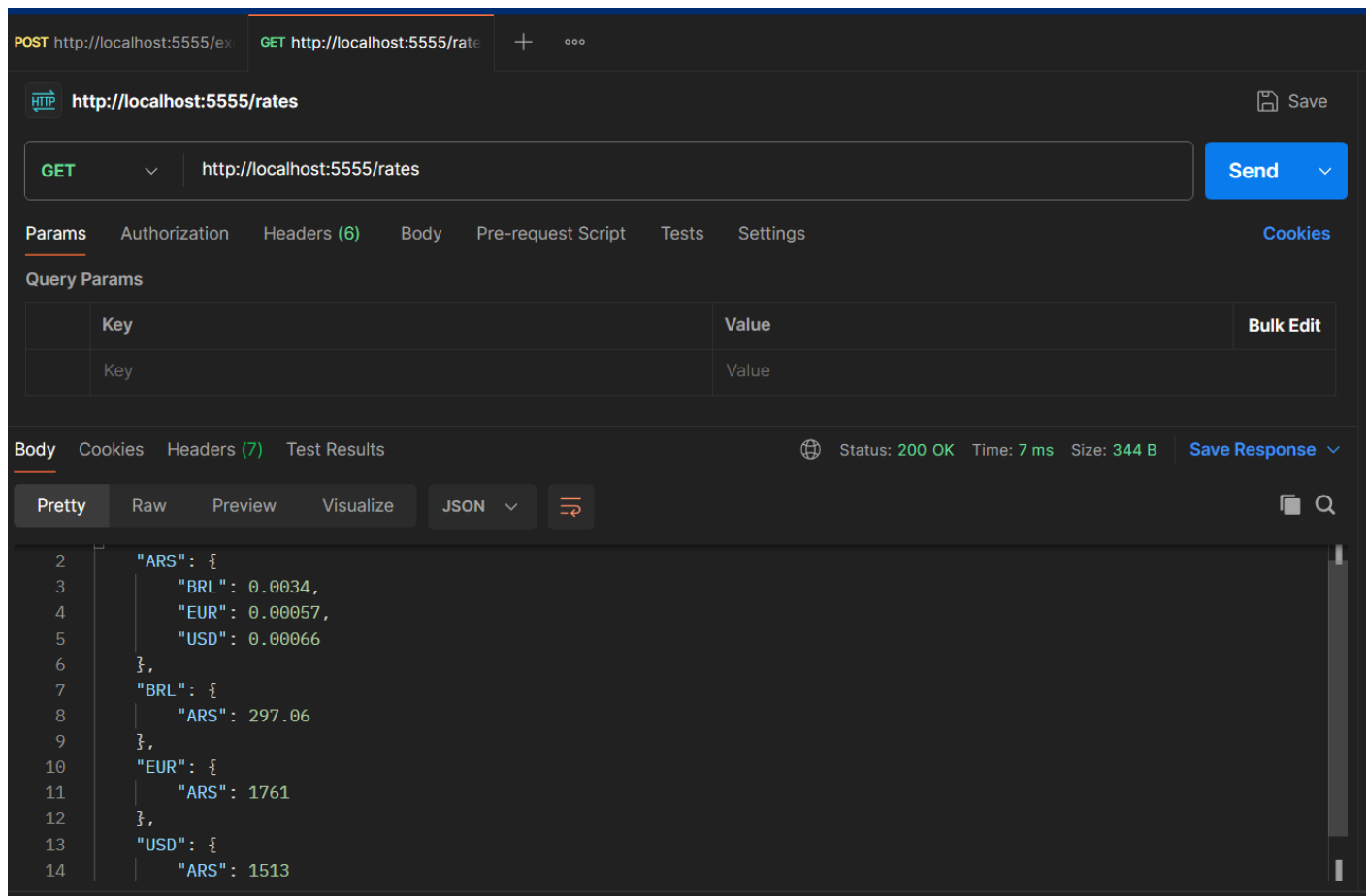
Figura 68. La API continúa respondiendo luego de rechazar la request inválida.
