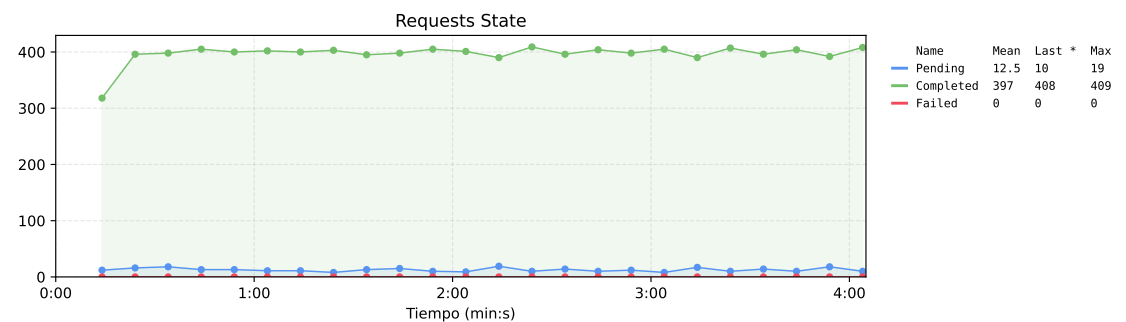
Figura 137. Estado de las requests de la propuesta 1.
