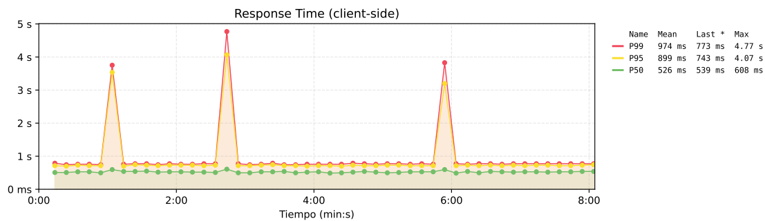
Figura 196. Tiempo de respuesta de la propuesta 2.
