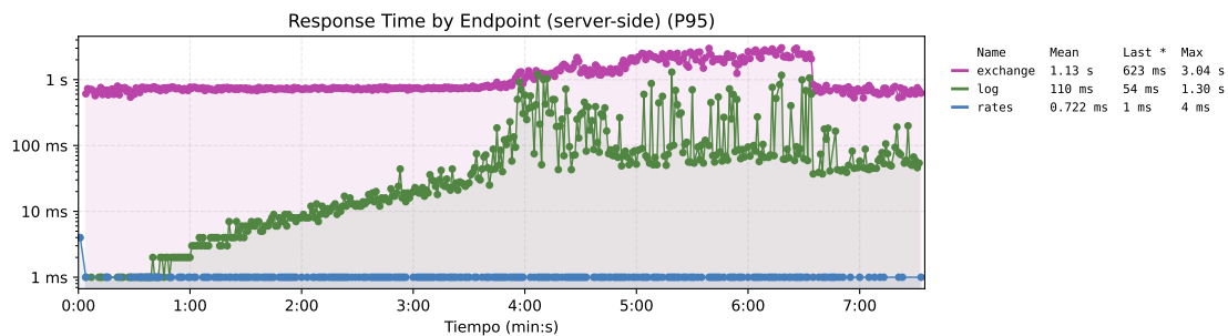
Figura 103. Tiempo de respuesta por endpoint del sistema base. El eje tiene una escala logarítmica.
