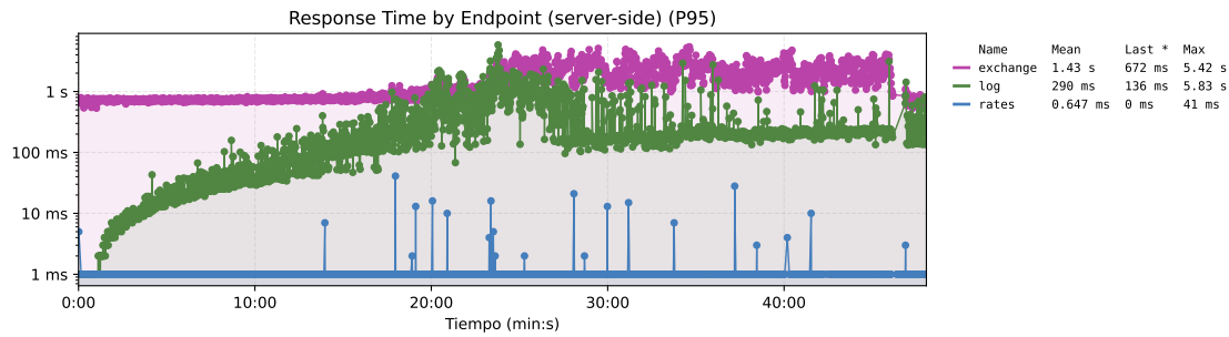
Figura 190. Tiempo de respuesta por endpoint de la propuesta 2. El eje tiene una escala logarítmica.
