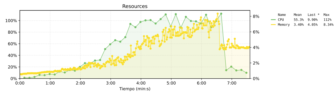
Figura 209. Estado de los recursos de la propuesta 3. El eje izquierdo muestra el uso de CPU, el eje derecho muestra el uso de memoria.
