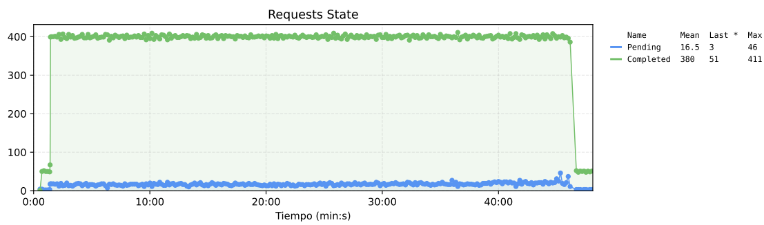
Figura 159. Estado de las requests de la propuesta 1.
