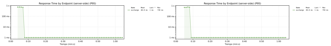
Figura 82. Comparativa de los resultados de latencia por endpoint entre la propuesta 3 (izquierda) y el sistema base (derecha) frente al escenario de concurrencia. Tanto las request aprobadas para la transferencia como las denegadas/falladas muestran tiempos iguales, lo que resulta en promedio de respuestas prácticamente iguales.
