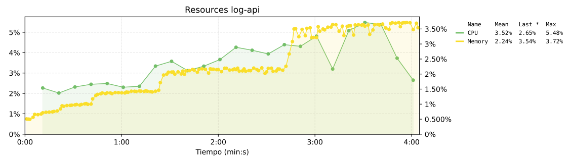
Figura 145. Estado de los recursos del nodo de logs de la propuesta 1. El eje izquierdo muestra el uso de CPU, el eje derecho muestra el uso de memoria.
