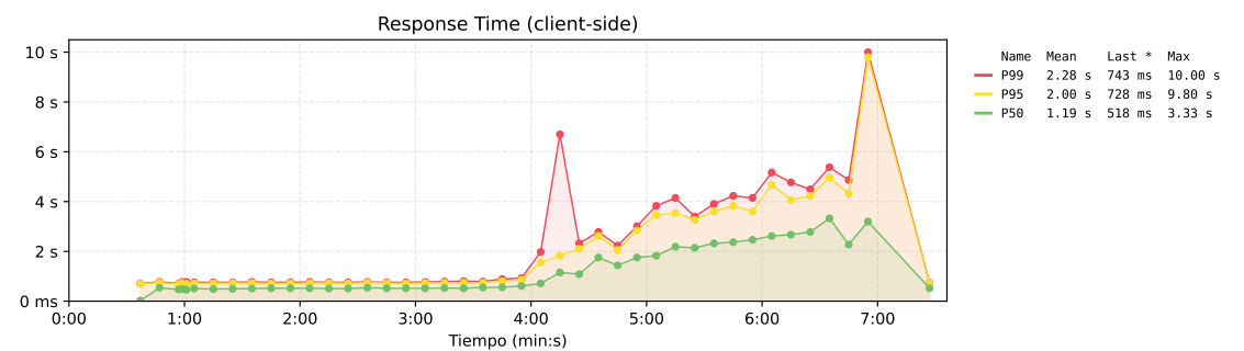
Figura 205. Tiempo de respuesta de la propuesta 3.
