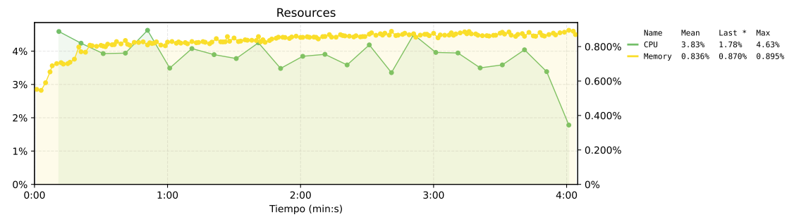
Figura 143. Estado de los recursos del nodo de exchange de la propuesta 1. El eje izquierdo muestra el uso de CPU, el eje derecho muestra el uso de memoria.
