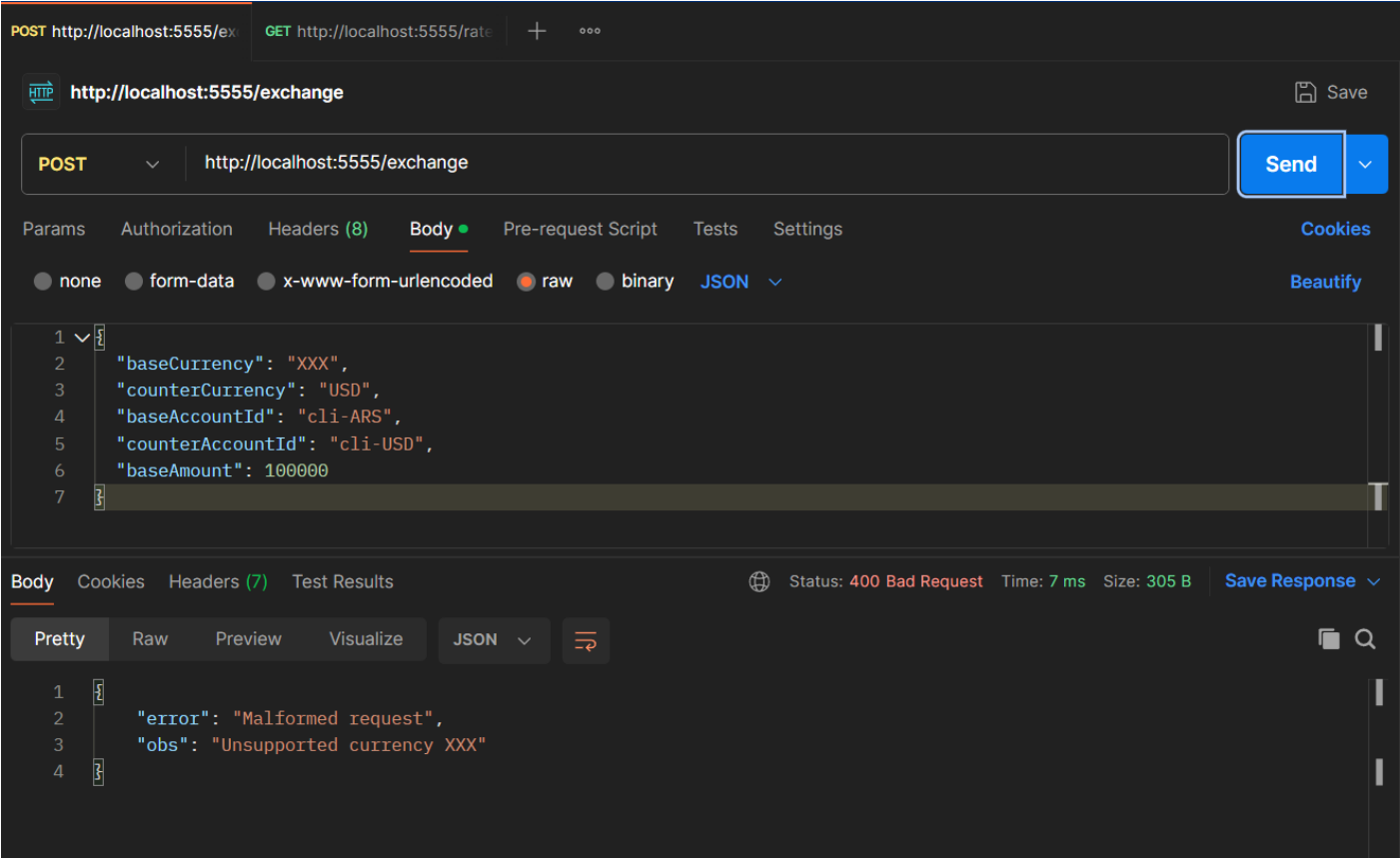
Figura 67. La propuesta 3 rechaza con HTTP 400 una moneda no soportada.
