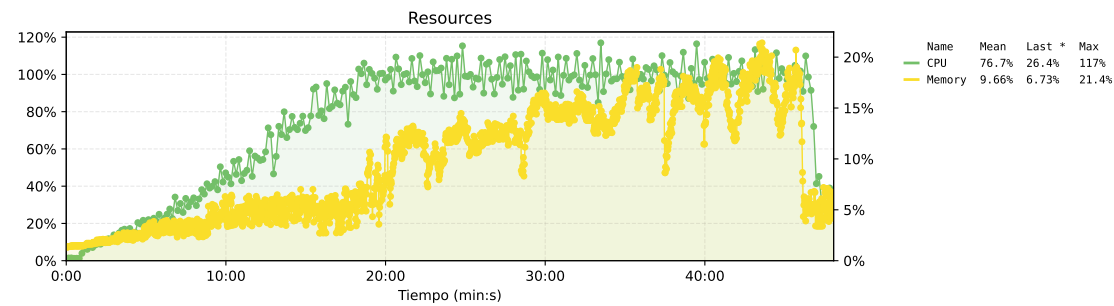
Figura 223. Estado de los recursos de la propuesta 3. El eje izquierdo muestra el uso de CPU, el eje derecho muestra el uso de memoria.
