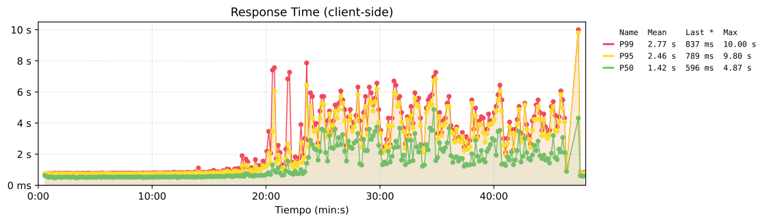
Figura 189. Tiempo de respuesta de la propuesta 2.
