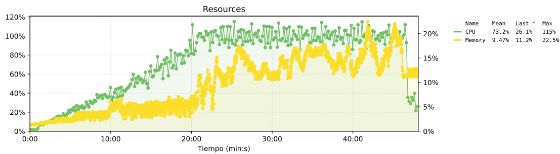
Figura 111. Estado de los recursos del sistema base. El eje izquierdo muestra el uso de CPU, el eje derecho muestra el uso de memoria.
