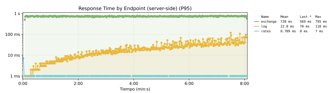
Figura 235. Tiempo de respuesta por endpoint de la propuesta 3. El eje tiene una escala logarítmica.
