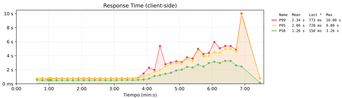
Figura 182. Tiempo de respuesta de la propuesta 2.
