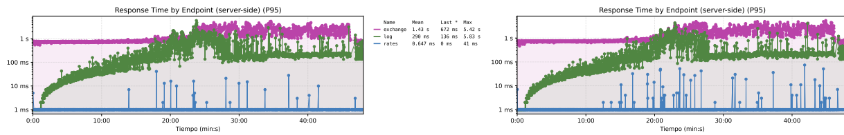
Figura 56. Comparativa de los resultados de latencia por endpoint entre la propuesta 2 (izquierda) y el sistema base (derecha) frente a un escenario de resistencia. En ambos casos el tiempo de respuesta de /log crece durante toda la prueba y arrastra a /exchange, que supera 1s a partir del minuto 20.
