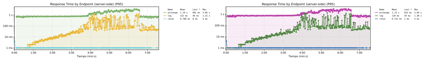
Figura 69. Comparativa de los resultados de latencia por endpoint entre la propuesta 3 (izquierda) y el sistema base (derecha) frente a un escenario de estrés. Se observan los mismos y ya conocidos problemas de degradación por el endpoint /log. Esperable ya que no es un problema que la propuesta busque resolver.
