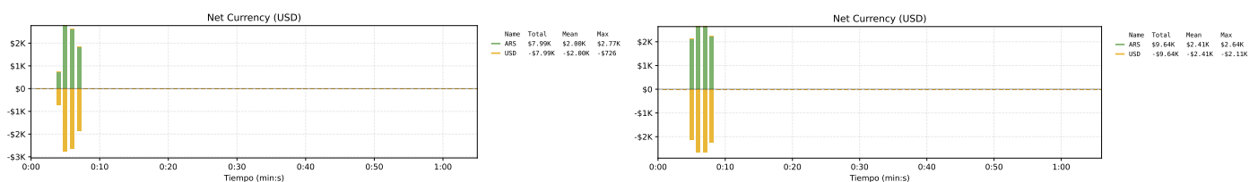
Figura 85. Comparativa de los resultados de volumen neto operado en cada moneda entre la propuesta 3 (izquierda) y el sistema base (derecha) frente al escenario de concurrencia. Análogamente a las métricas de volumen, se observa que la propuesta limitó el saldo operado a 7.99K es decir, dentro del saldo de 8K.
