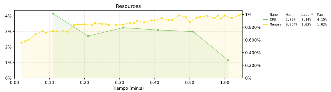
Figura 251. Estado de los recursos de la propuesta 3. El eje izquierdo muestra el uso de CPU, el eje derecho muestra el uso de memoria.
