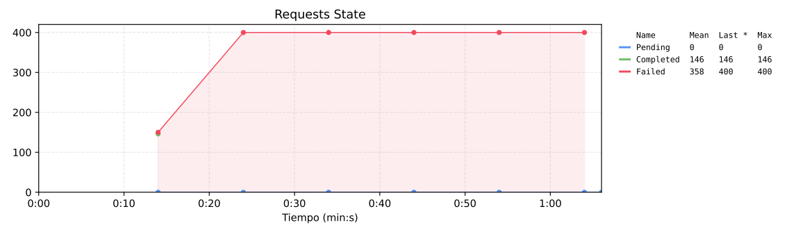
Figura 123. Estado de las requests del sistema base.
