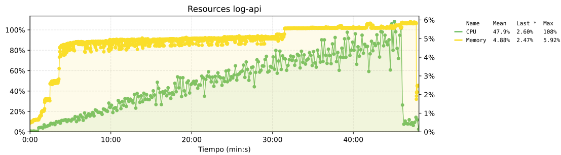
Figura 163. Estado de los recursos del nodo de logs de la propuesta 1. El eje izquierdo muestra el uso de CPU, el eje derecho muestra el uso de memoria.
