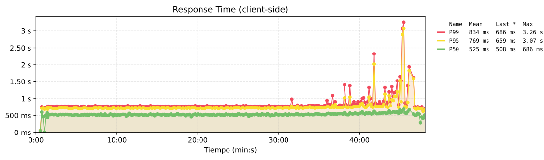
Figura 160. Tiempo de respuesta de la propuesta 1.
