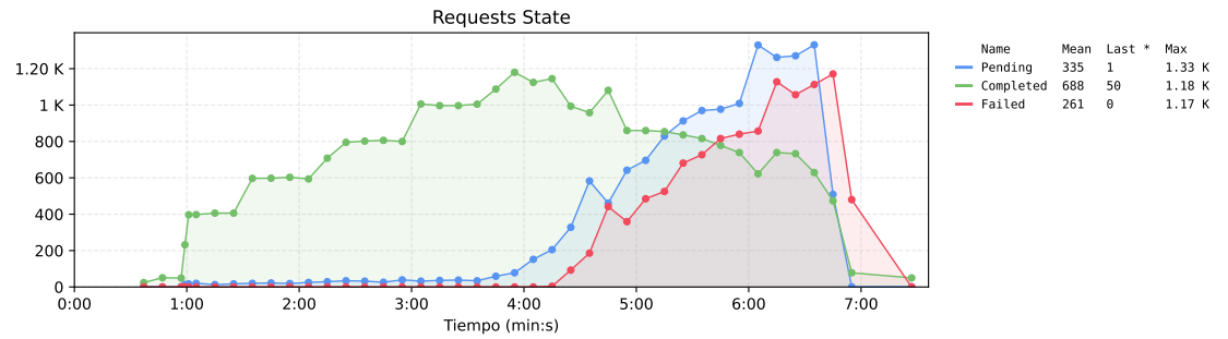
Figura 203. Estado de las requests de la propuesta 3.
