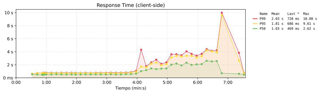
Figura 102. Tiempo de respuesta del sistema base.
