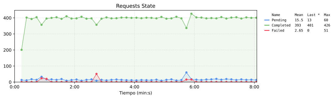
Figura 195. Estado de las requests de la propuesta 2.
