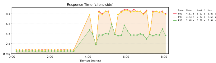
Figura 25. Posterior a la caída se observa el aumento en los tiempos de respuesta siendo estas devueltas por nginx como errores 502 en lugar de por el propio servidor.
