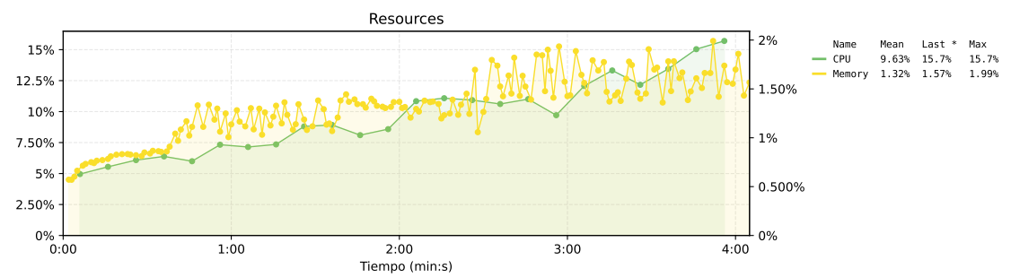
Figura 174. Estado de los recursos de la propuesta 2. El eje izquierdo muestra el uso de CPU, el eje derecho muestra el uso de memoria.
