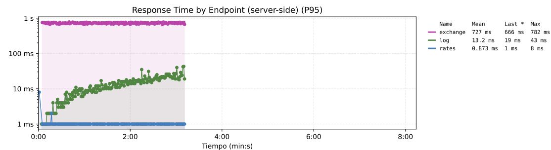
Figura 117. Tiempo de respuesta por endpoint del sistema base. El eje tiene una escala logarítmica.
