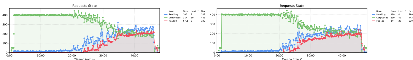
Figura 54. Comparativa de la disponibilidad ofrecida por la propuesta 2 (izquierda) y el sistema base (derecha) frente a un escenario de resistencia. Ambos sistemas comienzan a degradarse cerca del minuto 20 y hacia el minuto 35 alcanzan el mismo nivel de fallas. El promedio de respuestas satisfactorias por ventana es prácticamente el mismo (317 frente a 310). La propuesta 2 no mejora la disponibilidad frente a la degradación progresiva.
