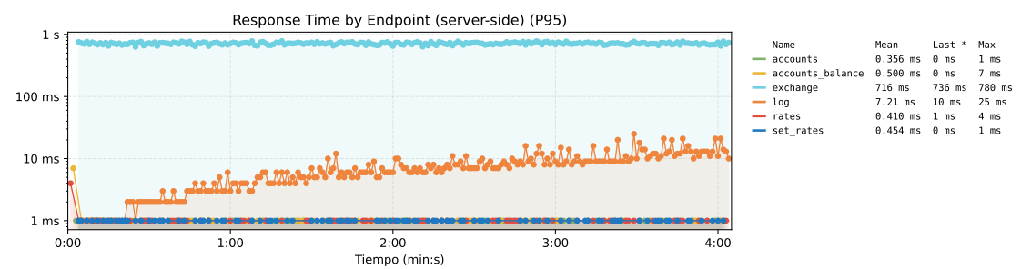
Figura 172. Tiempo de respuesta por endpoint de la propuesta 2. El eje tiene una escala logarítmica.
