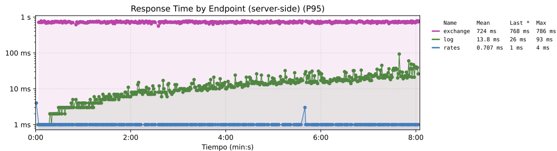
Figura 197. Tiempo de respuesta por endpoint de la propuesta 2. El eje tiene una escala logarítmica.
