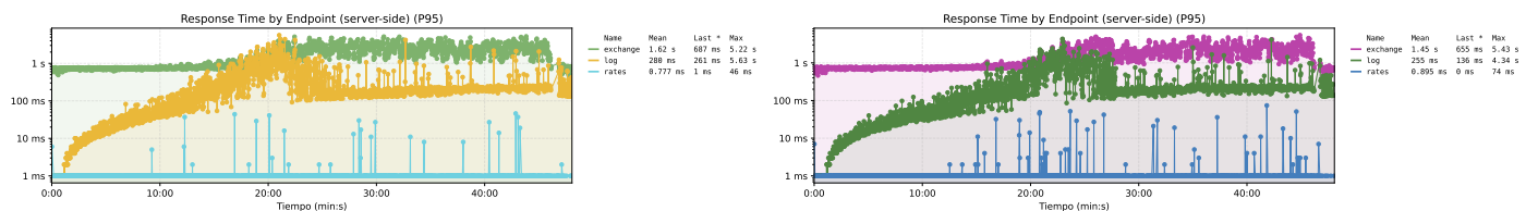
Figura 72. Comparativa de los resultados de latencia por endpoint entre la propuesta 3 (izquierda) y el sistema base (derecha) frente a un escenario de resistencia. Al igual como mencionamos en las pruebas de estrés, la situación no mejora con respecto a la degradación producida por el endpoint /log, esta vez, a lo largo del tiempo.
