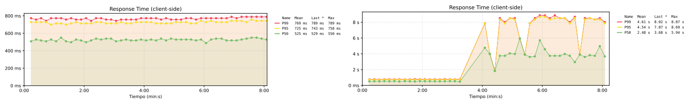
Figura 75. Comparativa de los resultados de latencia entre la propuesta 3 (izquierda) y el sistema base (derecha) frente a un escenario de caos. Tener cuidado con la visualización con respecto a los ejes. Los resultados de la propuesta 3 son todos tiempos irrisorios de 800ms frente a los 8s de timeout del sistema una vez este se caído.
