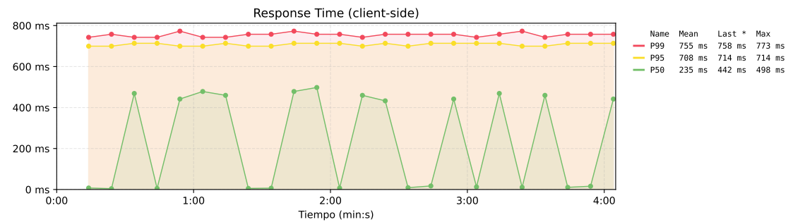
Figura 139. Tiempo de respuesta de la propuesta 1.
