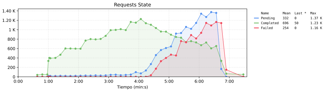
Figura 181. Estado de las requests de la propuesta 2.
