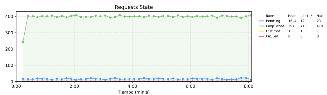
Figura 231. Estado de las requests de la propuesta 3.
