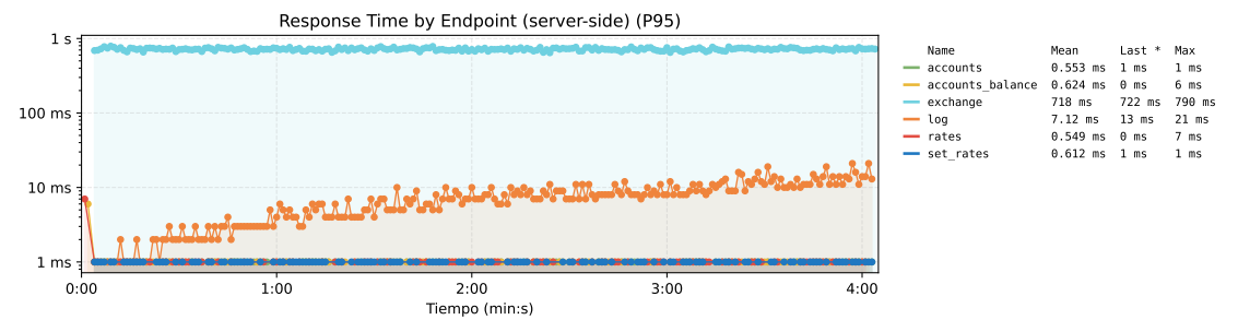
Figura 92. Tiempo de respuesta por endpoint del sistema base. El eje tiene una escala logarítmica.
