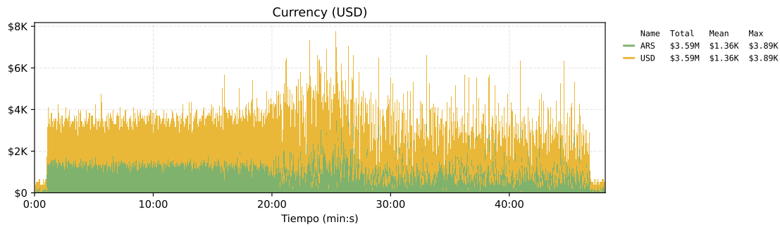
Figura 112. Volumen operado en cada moneda en el sistema base.
