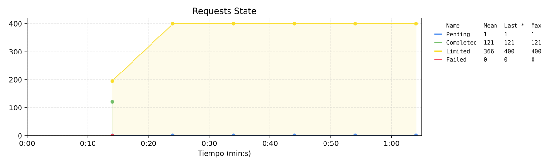
Figura 245. Estado de las requests de la propuesta 3.
