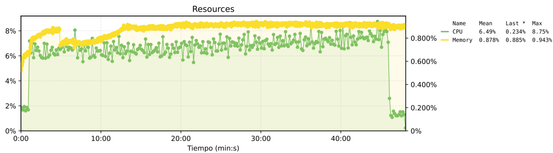
Figura 162. Estado de los recursos del nodo de exchange de la propuesta 1. El eje izquierdo muestra el uso de CPU, el eje derecho muestra el uso de memoria.
