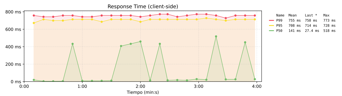
Figura 170. Tiempo de respuesta de la propuesta 2.
