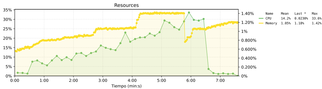
Figura 154. Estado de los recursos del nodo de exchange de la propuesta 1. El eje izquierdo muestra el uso de CPU, el eje derecho muestra el uso de memoria.
