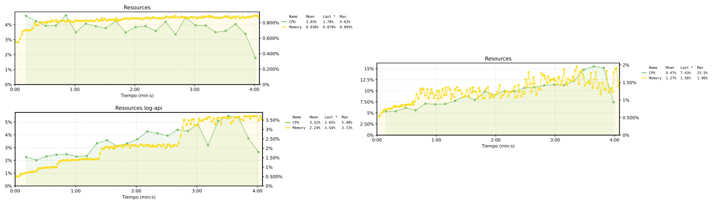
Figura 32. Comparativa del uso de recursos entre la propuesta 1 (izquierda, arriba la API de exchange y abajo el nodo de logs) y el sistema base (derecha) frente al escenario de carga. La API de exchange reduce su CPU promedio del 9.47 % al 3.83 %, y el consumo sumado de ambos nodos (7.35 %) es menor que el del sistema base.
