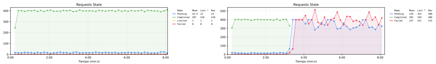
Figura 73. Comparativa de la disponibilidad ofrecida por la propuesta 3 (izquierda) y el sistema base (derecha) frente a un escenario de caos. La propuesta simplemente no falla ante las peticiones inválidas, permite al sistema seguir operando durante toda la prueba.
