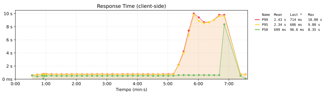
Figura 152. Tiempo de respuesta de la propuesta 1.
