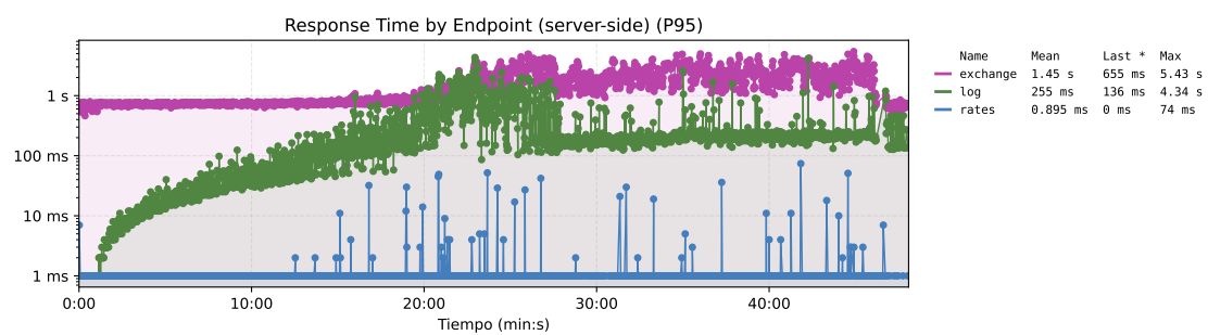
Figura 39. Tiempo de respuesta por endpoint del sistema base. El eje tiene una escala logarítmica.
