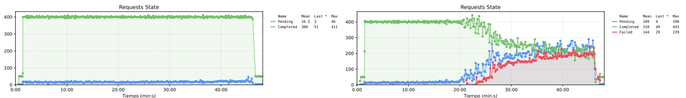
Figura 9. Comparativa de la disponibilidad ofrecida por la propuesta 1 (izquierda) y el sistema base (derecha) frente a un escenario de resistencia. El sistema base mostraba una degradación crítica a los 20 minutos, mientras que la propuesta 1 logra completar satisfactoriamente todas las request durante los 45 minutos.
