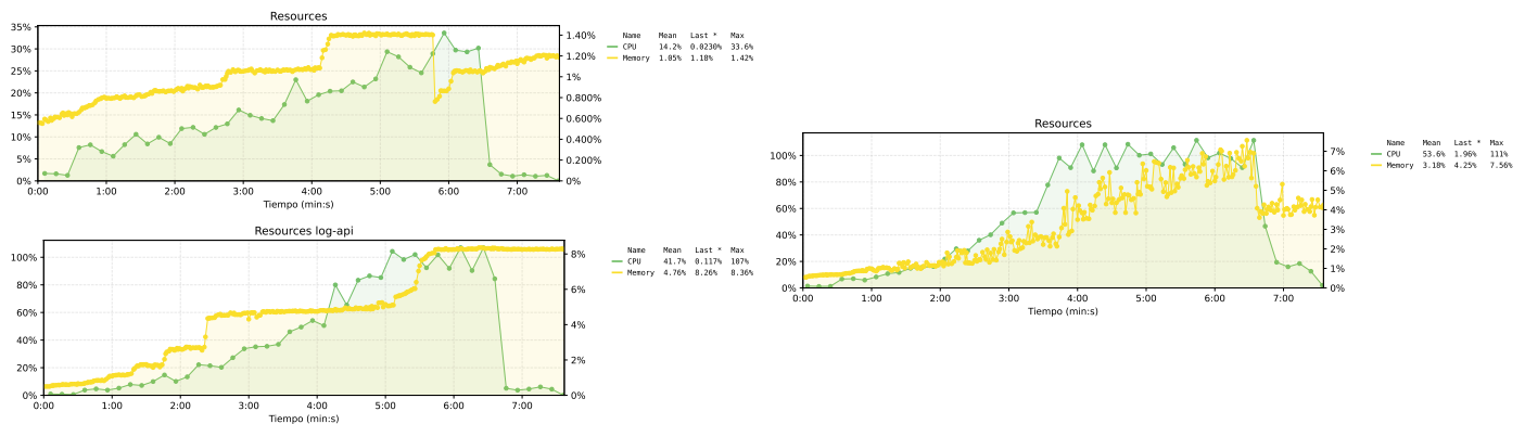
Figura 6. Comparativa de los resultados del uso de recursos entre la propuesta 1 (izquierda) y el sistema base (derecha) frente a un escenario de estrés. Destacar que consideramos la comparacion con respecto a ambos nodos, el nodo de exchange y el de logs. Se puede observar que el nodo de logs mantiene la carga con respecto a la del sistema base, incluso la aumenta. Esto es esperable con el aumento de la disponibilidad, mas request completadas implican mas entradas en el log. Sinembargo, el nodo de exchange apenas llevo a un 14.2 % de uso de CPU y 1.42 % de uso de memoria.
