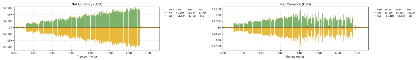
Figura 8. Comparativa de los resultados de volumen neto operado en cada moneda entre la propuesta 1 (izquierda) y el sistema base (derecha) frente a un escenario de estrés. Análogamente al volumen operado, se observa que el volumen neto también es mayor en la propuesta 1 frente al sistema base.
