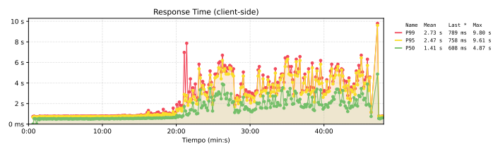
Figura 16. Se observa cómo nuevamente el aumento en la latencia desde la perspectiva del cliente es en el minuto 20, previo a la aparición de las primeras requests fallidas. Coherente con una degradación progresiva y no un error abrupto.
