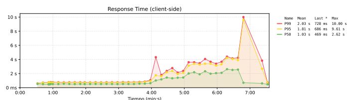
Figura 10. Se observa cómo previo a la pérdida de disponibilidad antes mencionada (4:30) el servidor ya empieza a presentar una degradación en los tiempos de respuesta desde el minuto 4.
