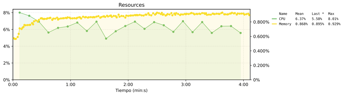
Figura 54. Estado de los recursos del nodo de exchange de la propuesta 1. El eje izquierdo muestra el uso de CPU, el eje derecho muestra el uso de memoria.
