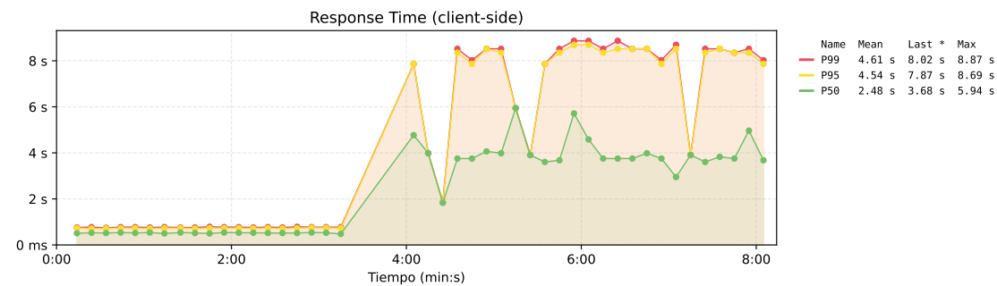
Figura 45. Tiempo de respuesta del sistema base.
