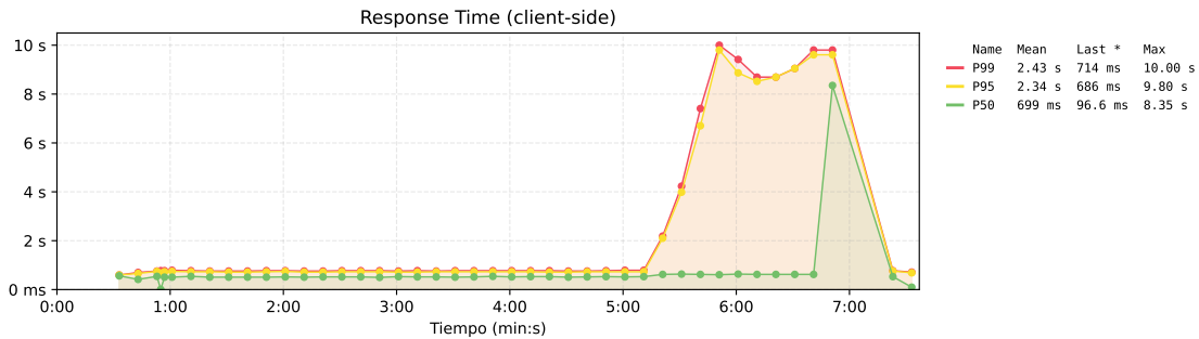
Figura 60. Tiempo de respuesta de la propuesta 1.
