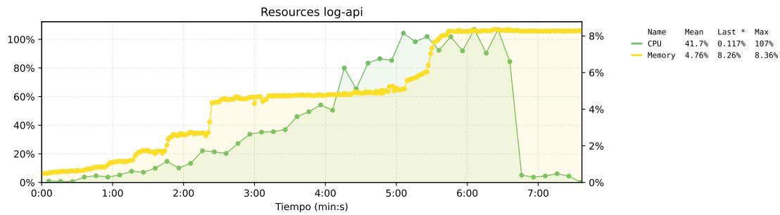
Figura 63. Estado de los recursos del nodo de logs de la propuesta 1. El eje izquierdo muestra el uso de CPU, el eje derecho muestra el uso de memoria.
