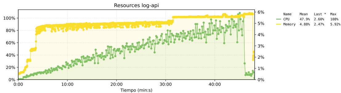
Figura 71. Estado de los recursos del nodo de logs de la propuesta 1. El eje izquierdo muestra el uso de CPU, el eje derecho muestra el uso de memoria.
