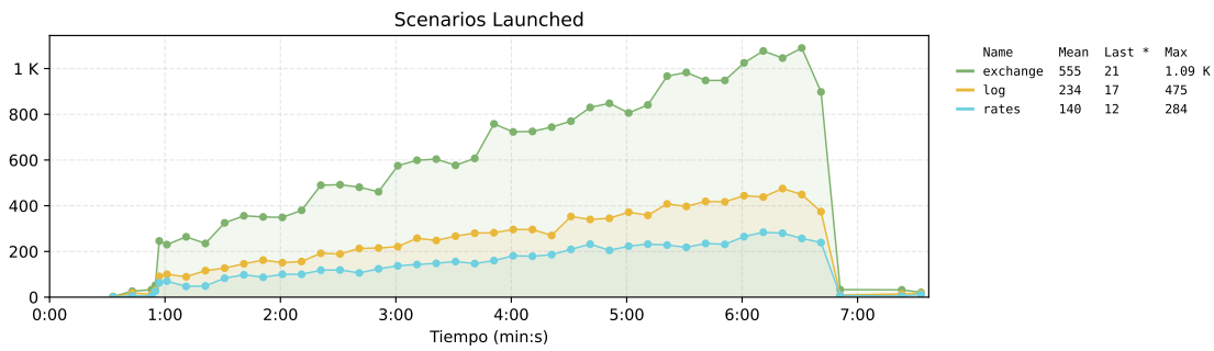
Figura 58. Escenarios de la propuesta 1.
