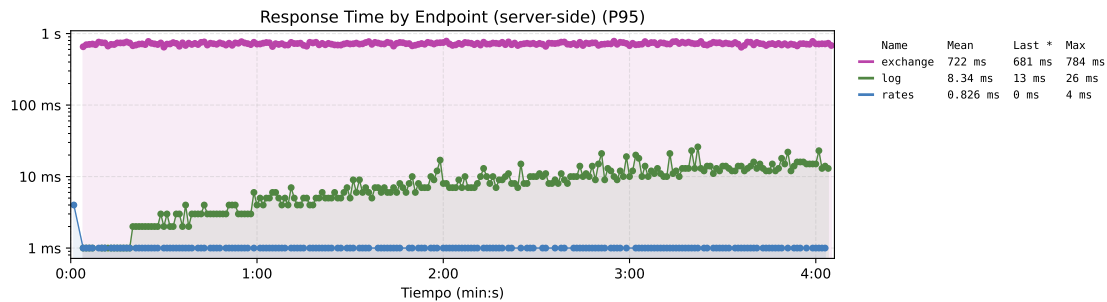
Figura 25. Tiempo de respuesta por endpoint del sistema base. El eje tiene una escala logaritmica.
