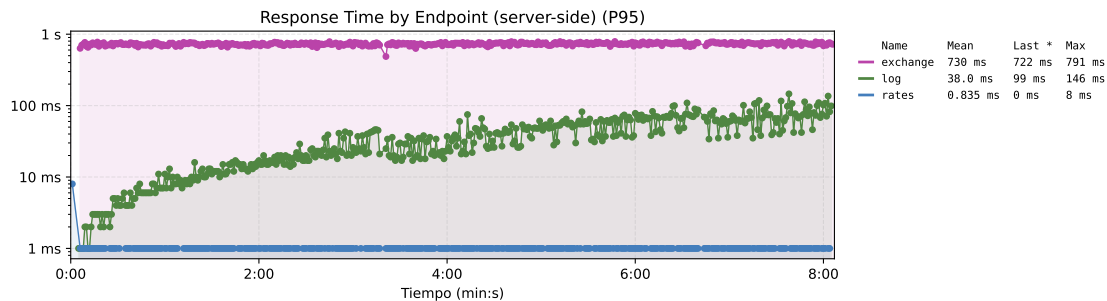
Figura 77. Tiempo de respuesta por endpoint de la propuesta 2. El eje tiene una escala logarítmica.
