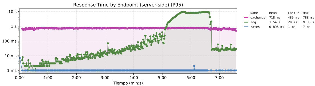
Figura 61. Tiempo de respuesta por endpoint de la propuesta 1. El eje tiene una escala logarítmica.
