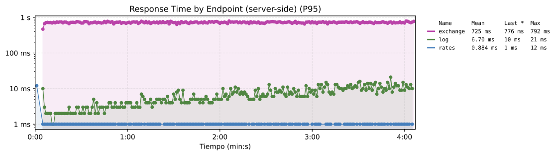
Figura 53. Tiempo de respuesta por endpoint de la propuesta 1. El eje tiene una escala logarítmica.
