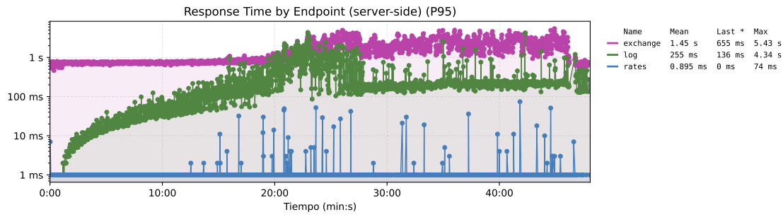
Figura 39. Tiempo de respuesta por endpoint del sistema base. El eje tiene una escala logaritmica.
