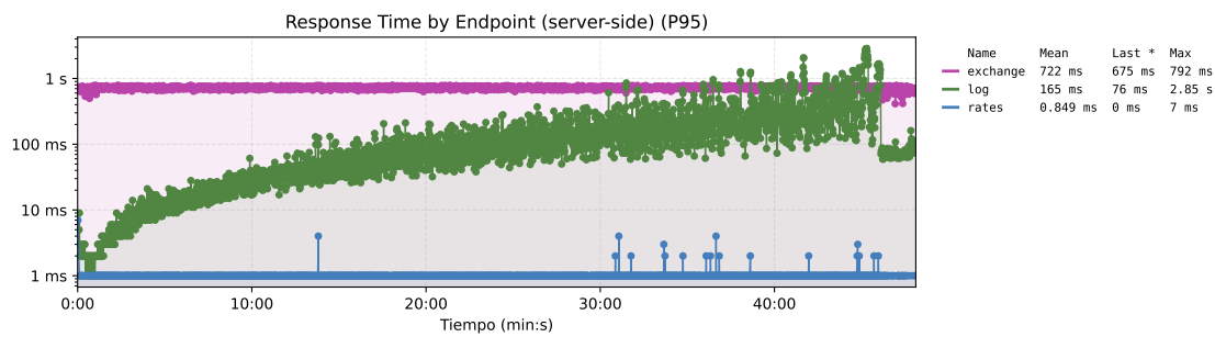
Figura 69. Tiempo de respuesta por endpoint de la propuesta 1. El eje tiene una escala logaritmica.
