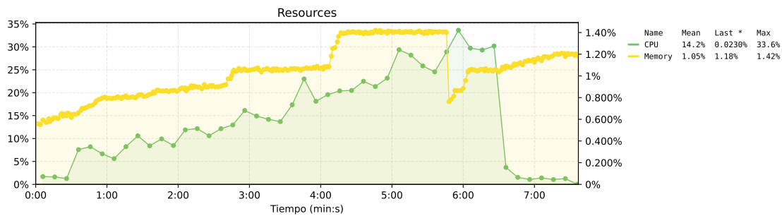
Figura 62. Estado de los recursos del nodo de exchange de la propuesta 1. El eje izquierdo muestra el uso de CPU, el eje derecho muestra el uso de memoria.
