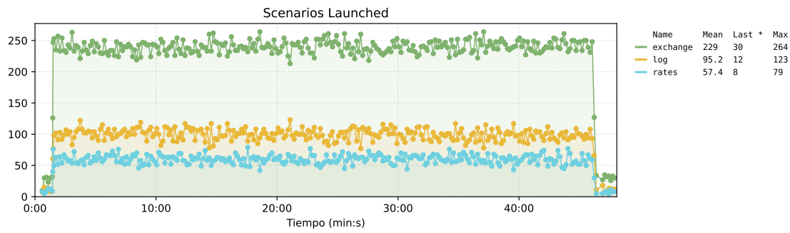
Figura 36. Escenarios del sistema base.
