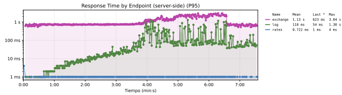
Figura 11. Se observa como el crecimiento en los tiempos de respuesta del log, dado por el crecimiento del mismo, impacta directamente en la latencia del endpoint de exchange.
