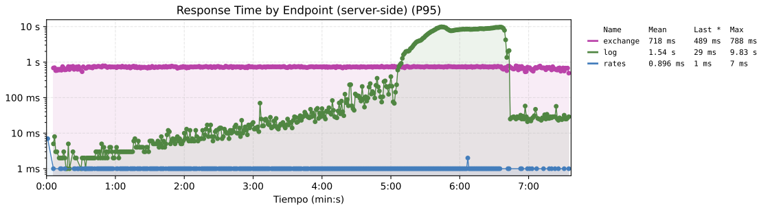
Figura 98. Tiempo de respuesta por endpoint de la propuesta 1. El eje tiene una escala logaritmica.
