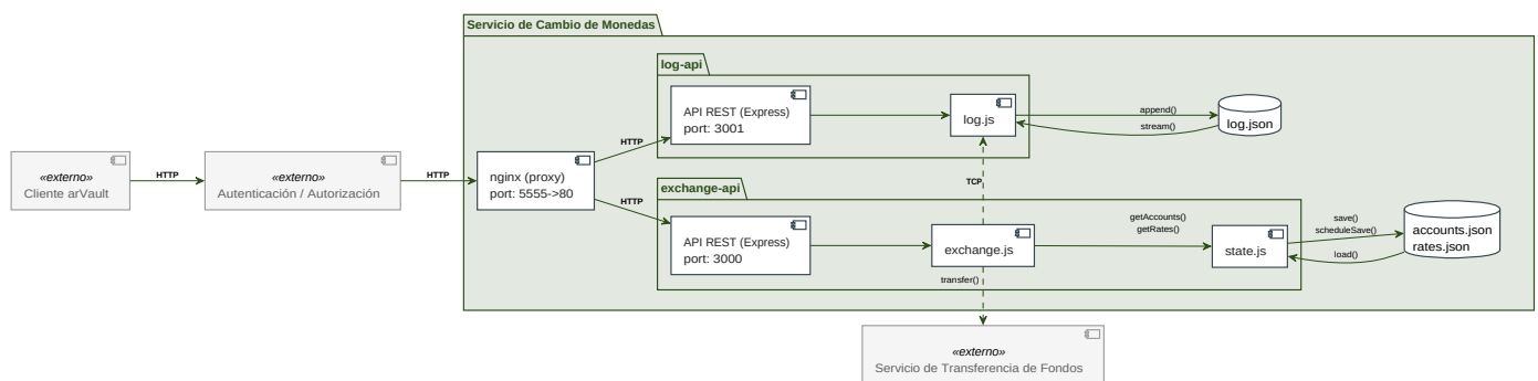
Figura 27. Diagrama Components & Connectors de la propuesta 1.
