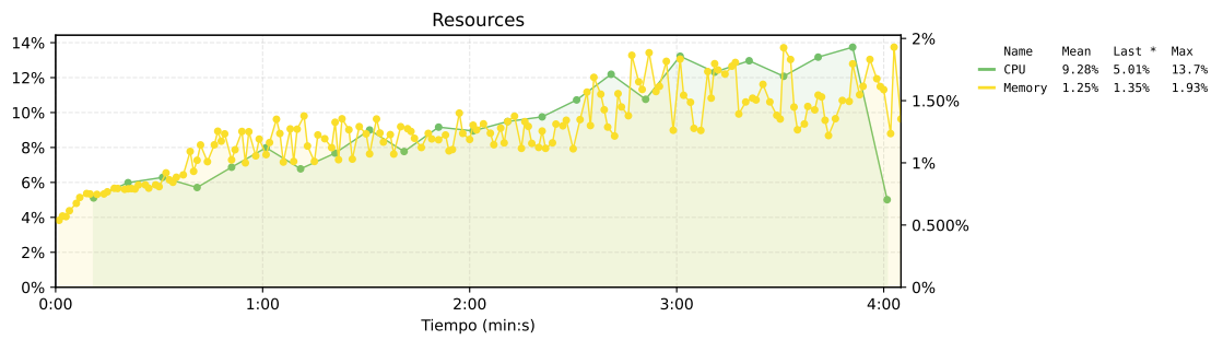
Figura 63. Estado de los recursos del sistema base. El eje izquierdo muestra el uso de CPU, el eje derecho muestra el uso de memoria.
