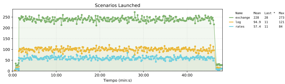
Figura 103. Escenarios de la propuesta 1.
