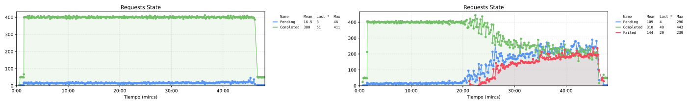
Figura 34. Comparativa de la disponibilidad ofrecida por la propuesta 1 (izquierda) y el sistema base (derecha) frente a un escenario de resistencia. El sistema base mostraba una degradación crítica a los 20 minutos, mientras que la propuesta 1 logro completar satisfactoriamente todas las request durante los 45 minutos.
