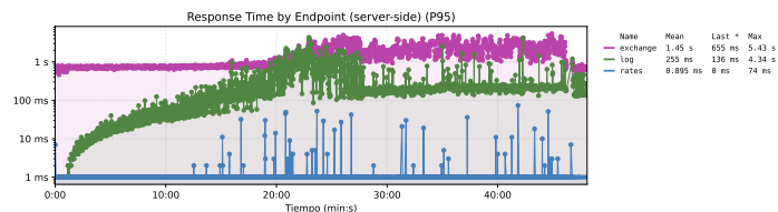
Figura 17. En cuanto a la latencia por endpoint se observan los mismo síntomas que los descritos en la prueba de estrés. El endpoint de log perjudica la latencia del endpoint de exchange conforme el tamaño del log aumenta y con este su tiempo de respuesta. Este comportamiento se evidencia a partir del minuto 20, consistente con las conclusiones de disponibilidad y latencia antes mencionadas.
