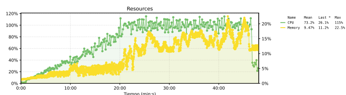
Figura 18. Se observa un incremento en el uso de recursos, especialmente de CPU, alcanzando este el máximo disponible a los 20 minutos. El uso de memoria también siguió incrementando con respecto a las observaciones en las pruebas de carga, llegando hasta un máximo de 22.5 % de la memoria disponible.
