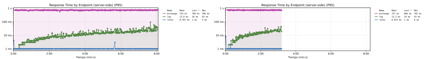
Figura 55. Comparativa de los resultados de latencia por endpoint entre la propuesta 2 (izquierda) y el sistema base (derecha) frente a un escenario de caos. A diferencia del sistema base, en la propuesta 2 las métricas del servidor se siguen reportando durante toda la prueba, ya que el proceso que las emite vuelve a estar disponible. El tiempo de respuesta de /log sigue creciendo después de cada reinicio en lugar de volver a su valor inicial, lo que evidencia que el estado persistido en disco se conserva entre reinicios.
