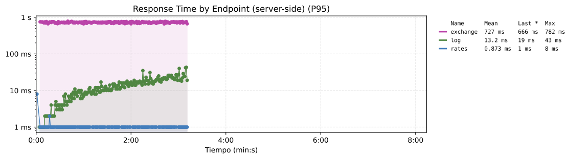
Figura 83. Tiempo de respuesta por endpoint del sistema base. El eje tiene una escala logaritmica.
