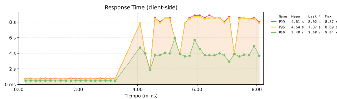
Figura 22. Posterior a la caída se observa el aumento en los tiempos de respuesta siendo estas devueltas por nginx como errores 502 en lugar de por el propio servidor.
