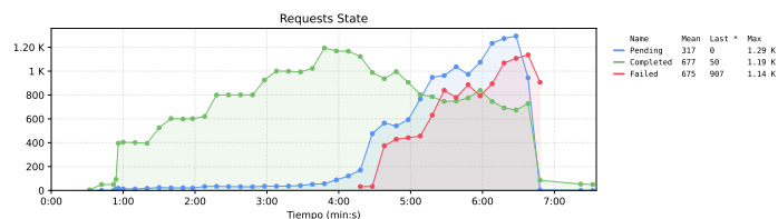
Figura 9. Se observa que el servidor bajo el crecimiento de la carga encuentra su punto de quiebre al rededor del minuto 4:30. A partir de ese momento, la disponibilidad del sistema se ve comprometida y se continuan compleando solicitudes pero otras fallan.
