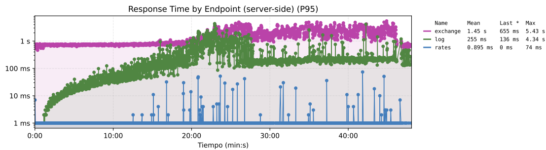
Figura 76. Tiempo de respuesta por endpoint del sistema base. El eje tiene una escala logaritmica.
