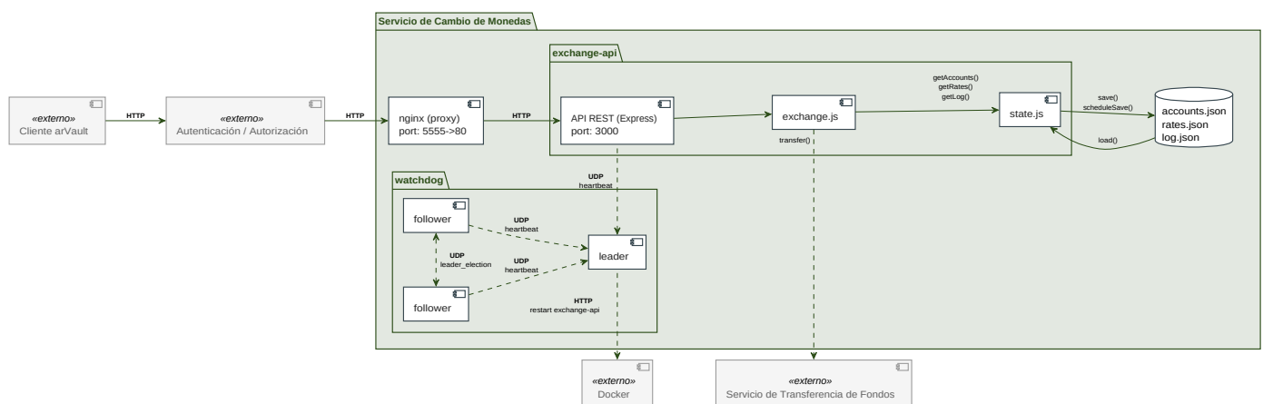
Figura 40. Diagrama Components & Connectors de la propuesta 2.
