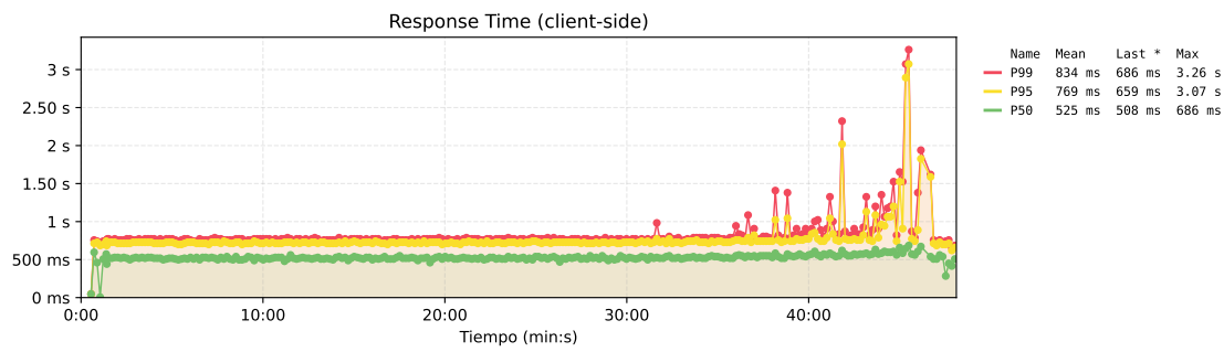
Figura 105. Tiempo de respuesta de la propuesta 1.
