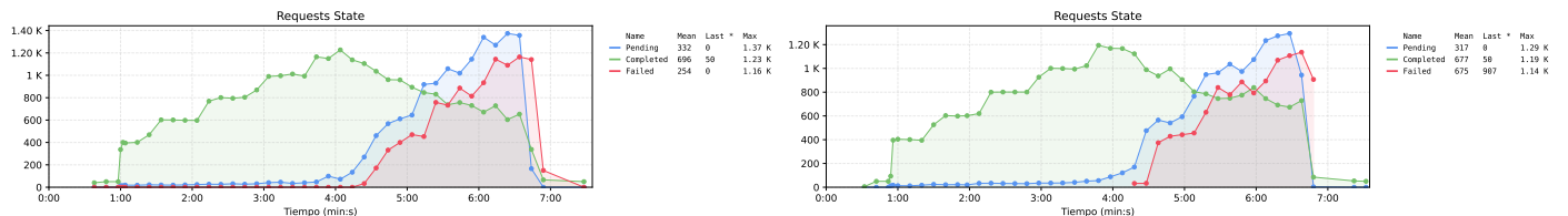
Figura 41. Comparativa de la disponibilidad ofrecida por la propuesta 2 (izquierda) y el sistema base (derecha) frente a un escenario de estrés. Ambos sistemas alcanzan su punto de quiebre en el mismo momento, alrededor del minuto 4:15, y presentan picos de fallas similares (1.16K frente a 1.14K por ventana). El promedio de respuestas satisfactorias es prácticamente el mismo (696 frente a 677). Como se esperaba, la táctica no mejora la disponibilidad frente a la sobrecarga.
