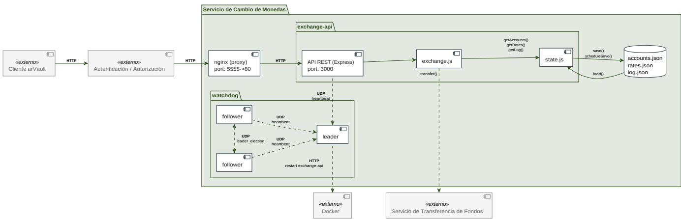
Figura 15. Diagrama Components & Connectors de la propuesta 2.
