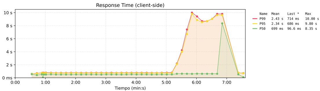
Figura 72. Tiempo de respuesta de la propuesta 1.
