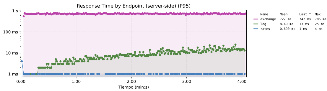
Figura 89. Tiempo de respuesta por endpoint de la propuesta 2. El eje tiene una escala logarítmica.
