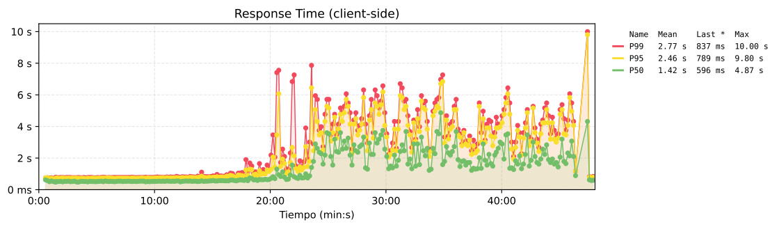
Figura 102. Tiempo de respuesta de la propuesta 2.
