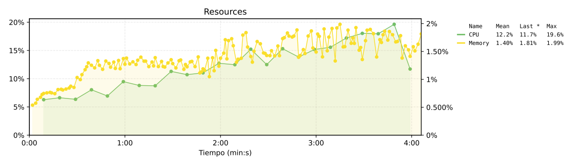
Figura 38. Estado de los recursos del sistema base. El eje izquierdo muestra el uso de CPU, el eje derecho muestra el uso de memoria.
