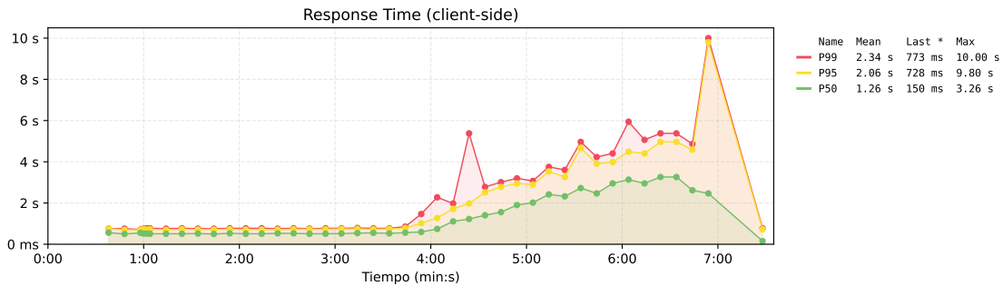
Figura 148. Tiempo de respuesta de la propuesta 2.
