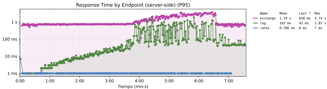
Figura 149. Tiempo de respuesta por endpoint de la propuesta 2. El eje tiene una escala logarítmica.
