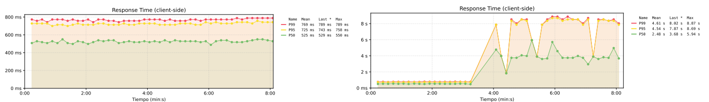
Figura 72. Comparativa de los resultados de latencia entre la propuesta 3 (izquierda) y el sistema base (derecha) frente a un escenario de caos.
