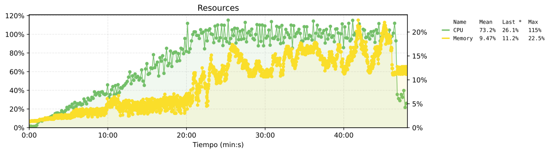
Figura 98. Estado de los recursos del sistema base. El eje izquierdo muestra el uso de CPU, el eje derecho muestra el uso de memoria.
