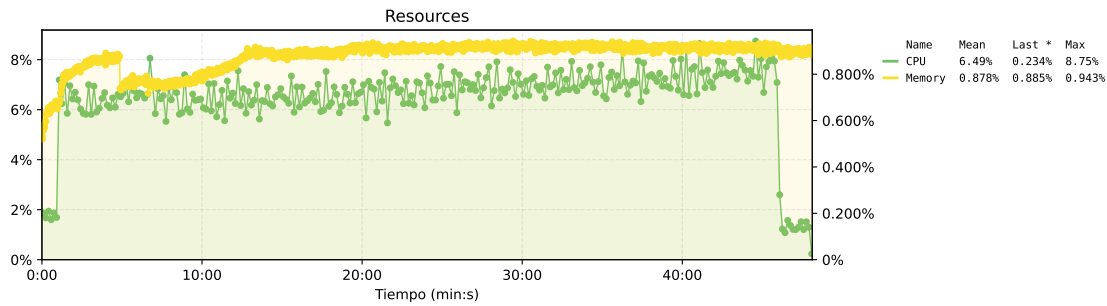
Figura 135. Estado de los recursos del nodo de exchange de la propuesta 1. El eje izquierdo muestra el uso de CPU, el eje derecho muestra el uso de memoria.
