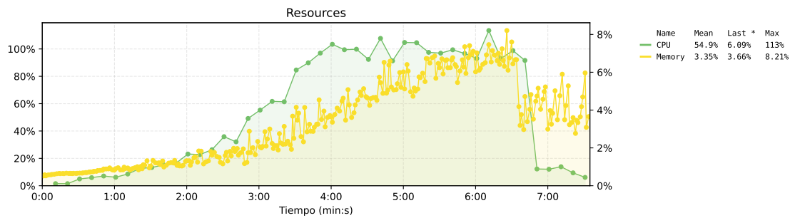
Figura 150. Estado de los recursos de la propuesta 2. El eje izquierdo muestra el uso de CPU, el eje derecho muestra el uso de memoria.
