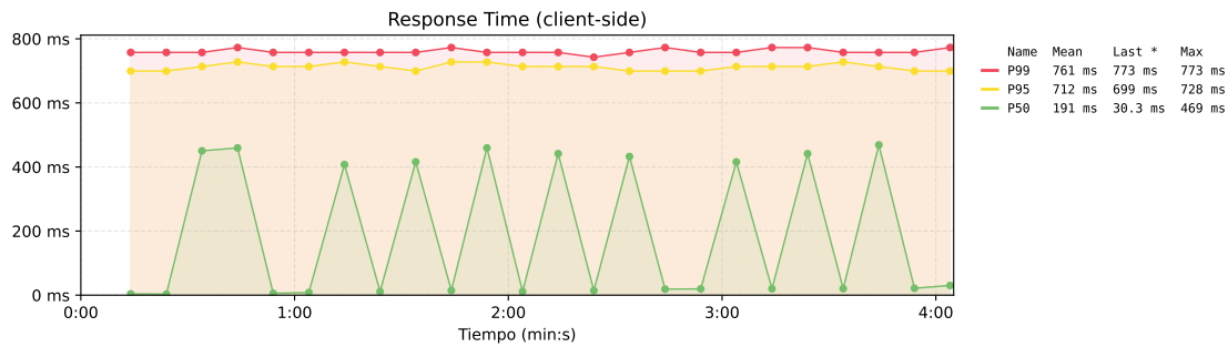
Figura 141. Tiempo de respuesta de la propuesta 2.
