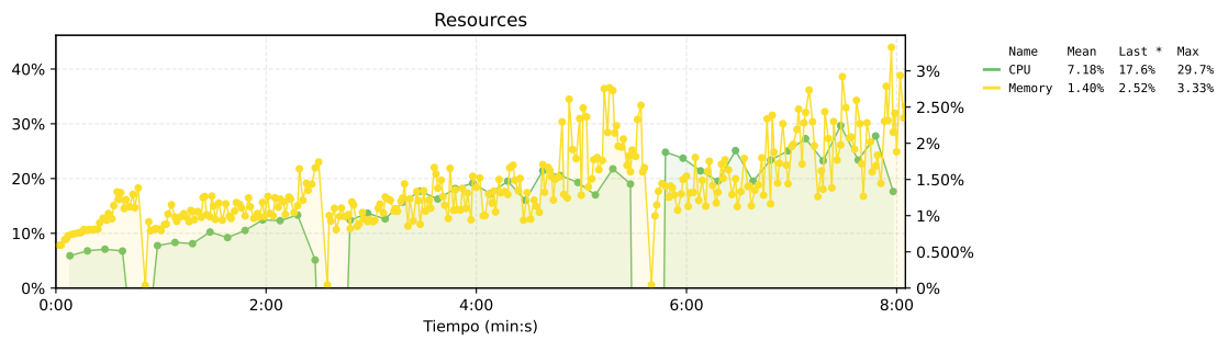
Figura 164. Estado de los recursos de la propuesta 2. El eje izquierdo muestra el uso de CPU, el eje derecho muestra el uso de memoria.
