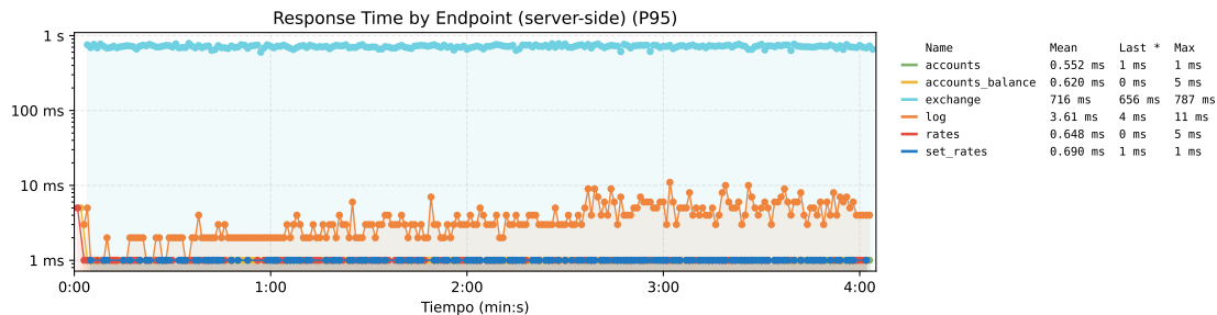
Figura 118. Tiempo de respuesta por endpoint de la propuesta 1. El eje tiene una escala logarítmica.
