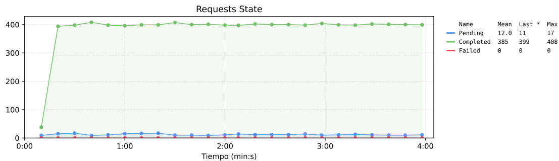
Figura 116. Estado de las requests de la propuesta 1.
