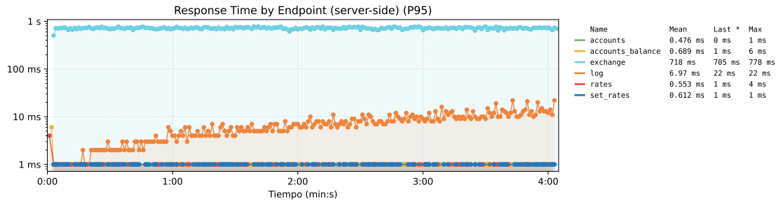
Figura 83. Tiempo de respuesta por endpoint del sistema base. El eje tiene una escala logarítmica.
