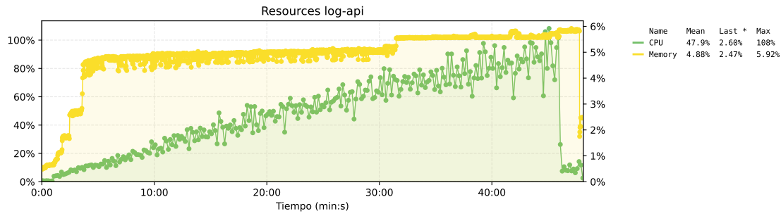
Figura 136. Estado de los recursos del nodo de logs de la propuesta 1. El eje izquierdo muestra el uso de CPU, el eje derecho muestra el uso de memoria.
