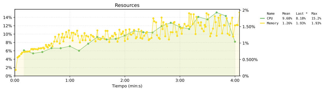
Figura 115. Estado de los recursos de la propuesta 2. El eje izquierdo muestra el uso de CPU, el eje derecho muestra el uso de memoria.
