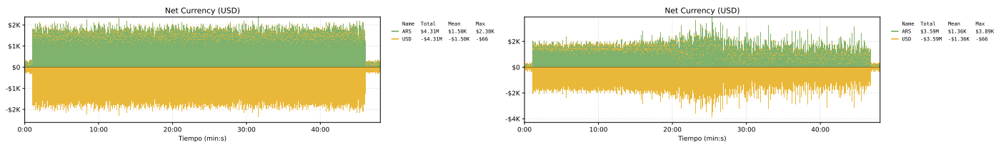
Figura 39. Comparativa de los resultados de volumen neto operado en cada moneda entre la propuesta 1 (izquierda) y el sistema base (derecha) frente a un escenario de resistencia. Análogamente al volumen operado, se observa que el volumen neto también es mayor en la propuesta 1 frente al sistema base en la misma proporción.
