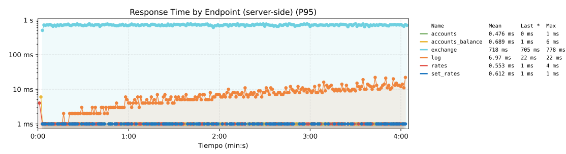
Figura 62. Tiempo de respuesta por endpoint del sistema base. El eje tiene una escala logarítmica.
