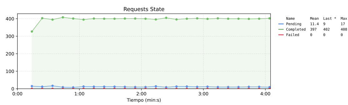
Figura 60. Estado de las requests del sistema base.
