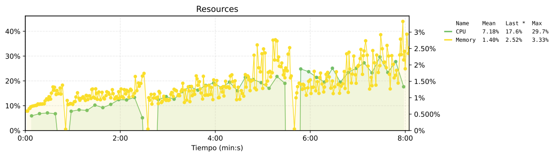
Figura 136. Estado de los recursos de la propuesta 2. El eje izquierdo muestra el uso de CPU, el eje derecho muestra el uso de memoria.
