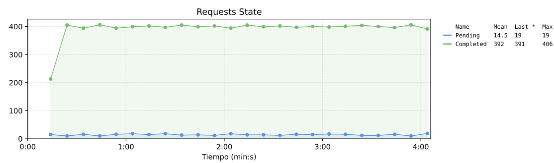
Figura 23. Estado de las requests del sistema base.
