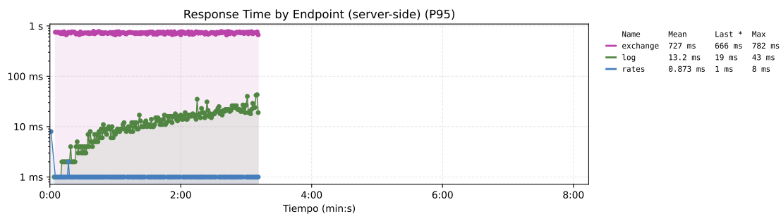
Figura 46. Tiempo de respuesta por endpoint del sistema base. El eje tiene una escala logarítmica.
