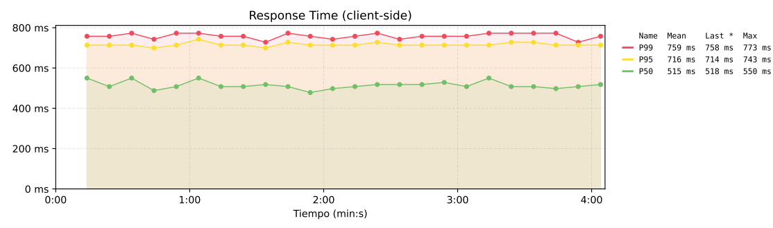
Figura 24. Tiempo de respuesta del sistema base.
