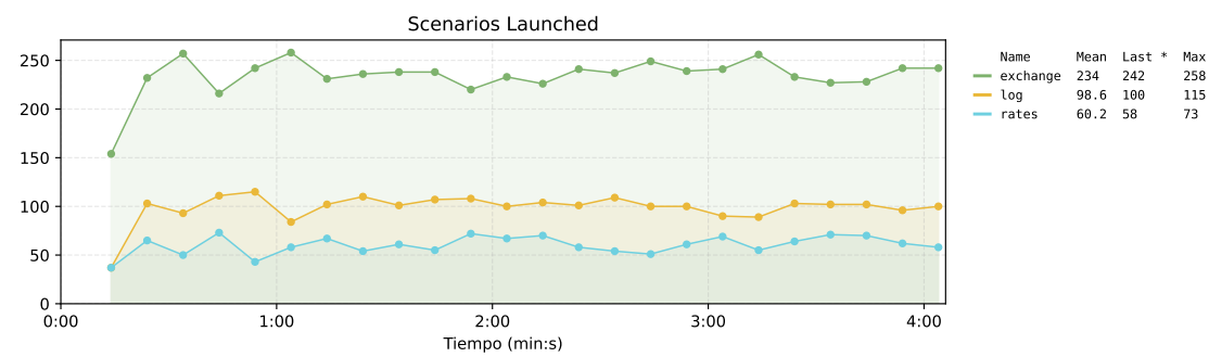
Figura 22. Escenarios del sistema base.
