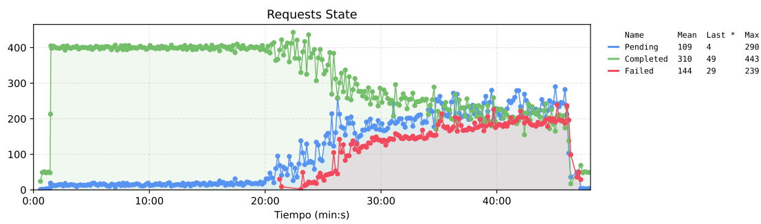
Figura 37. Estado de las requests del sistema base.
