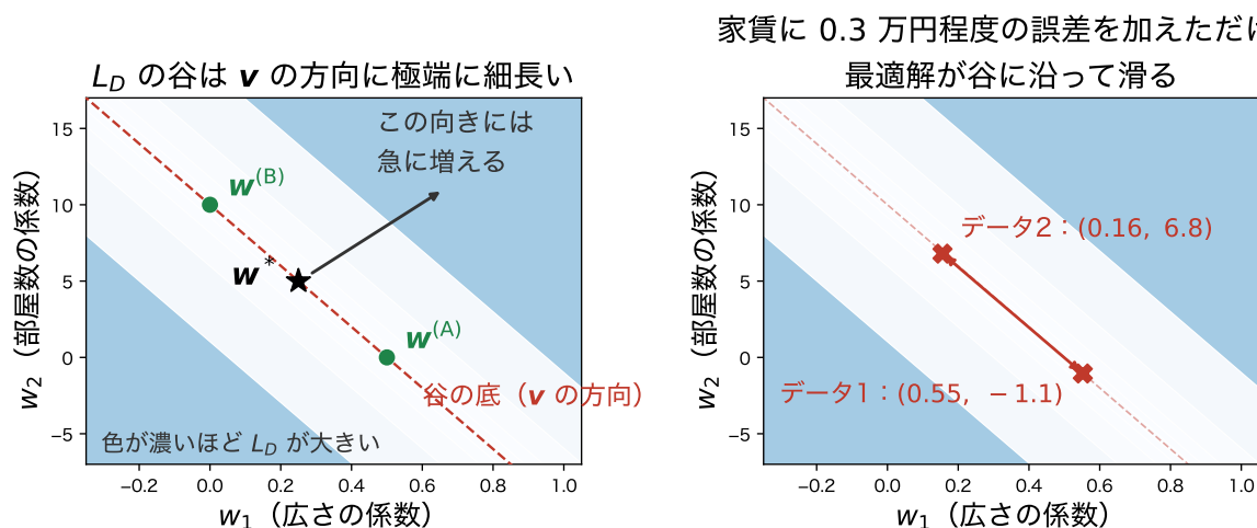
図 18 ほぼ平らな谷。左：経験損失 L_D の等高線。 \mathbf{v} = (0, 1, -20)^\top の方向にはほとんど増えず、それと交わる向きには急に増える。右：家賃に 0.3 万円程度の誤差を加えた 2 通りのデータについて最適解を求めたもの。谷に沿って大きく離れ、「広さ中心のモデル」と「部屋数中心のモデル」のどちらにもなりうる。なお縦軸と横軸で目盛りの刻みが異なるため、谷の細さは実際よりも緩やかに見えている。
