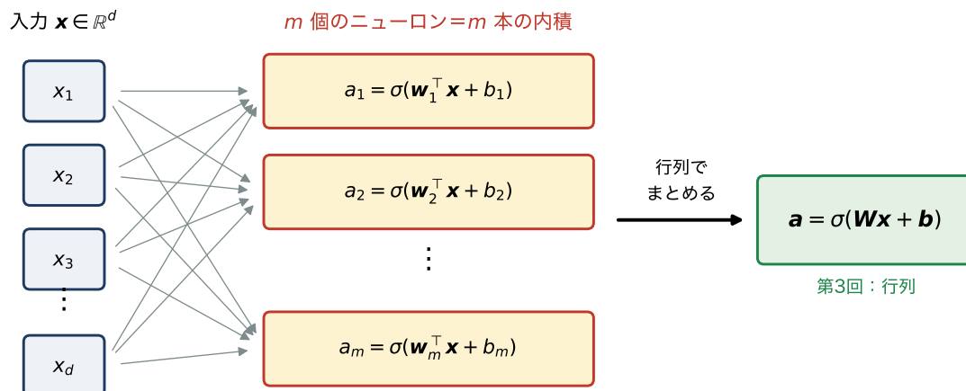
図 11 層は m 個のニューロンからなり、 m 本の内積を並べたものである。次回学ぶ行列を用いると、これは一つの式 \mathbf{a} = \sigma(\mathbf{W}\mathbf{x} + \mathbf{b}) にまとまる。
