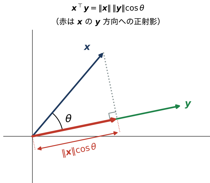
図4 内積の幾何学的意味。 \mathbf{x} を \mathbf{y} の方向に射影した長さ \|\mathbf{x}\| \cos \theta に、 \|\mathbf{y}\| を掛けたものが内積である。
