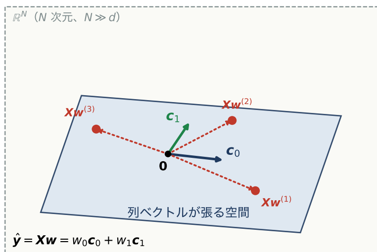
図 16 w を動かしたときの予測 \hat{y} = Xw の動く範囲。 w をどう選んでも \hat{y} は列ベクトルの張る部分空間から出られない。図は \text{rank}(X) = 2 の場合（平面）を描いた模式図である。
