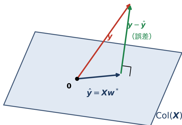
図 17 列空間と最小二乗法。予測 \mathbf{X}\mathbf{w} は列空間の中しか動けないため、誤差を最小にするのは \mathbf{y} を列空間へ正射影した点である。
