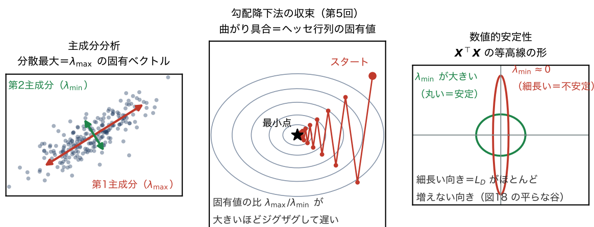
図 20 固有値が現れる 3 つの場面（概念図）。左：主成分分析。データが最も散らばる方向が共分散行列の最大固有値の固有ベクトルである。中：勾配降下法。等高線が細長い（固有値の比が大きい）ほど経路がジグザグし、収束が遅くなる。右：数値的安定性。 \mathbf{X}^\top \mathbf{X} の最小固有値が 0 に近いほど等高線が細長くなり、その向きには L_D がほとんど増えない。これが図 18 で見た「平らな谷」である。
