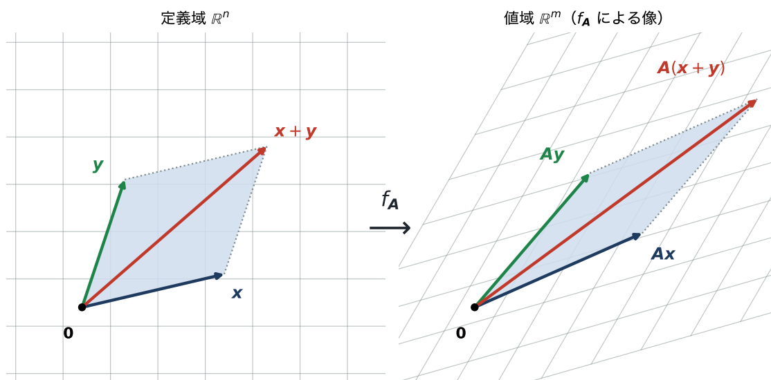
図 15 線形写像 f_A(x) = Ax のはたらき ( n = m = 2 の例)。格子は格子に、原点は原点に、平行四辺形は平行四辺形に写る。右図で Ax, Ay の作る平行四辺形の対角線が A(x+y) になっていることが、加法性に当たる。
