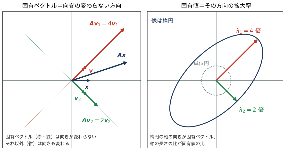
図 19 A = \begin{pmatrix} 3 & 1 \\ 1 & 3 \end{pmatrix} による変換。左: 固有ベクトル v_1, v_2 は向きが変わらず、長さだけがそれぞれ 4 倍、2 倍になる。固有ベクトルでない x は向きまで変わる。右: 単位円の像は楕円になり、楕円の軸の向きが固有ベクトル、軸の長さの比が固有値の比
