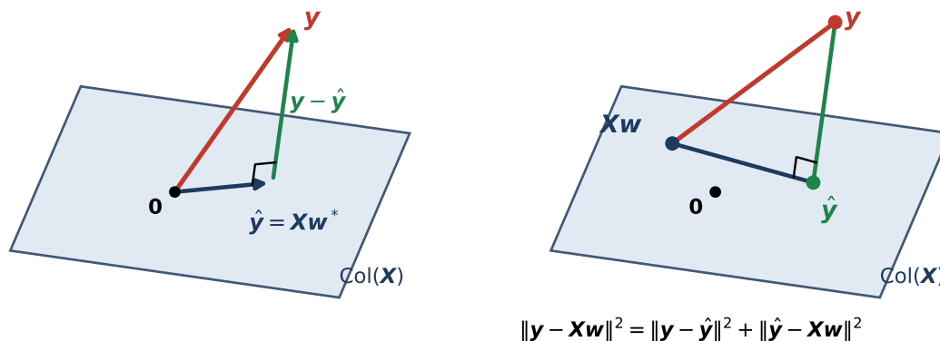
図 22 最小二乗法の幾何学。左：誤差 \mathbf{y} - \hat{\mathbf{y}} が列空間と直交する点が最良の予測である。右：列空間上の他の点 \mathbf{X}\mathbf{w} をとると、三平方の定理により \|\mathbf{y} - \mathbf{X}\mathbf{w}\|^2 = \|\mathbf{y} - \hat{\mathbf{y}}\|^2 + \|\hat{\mathbf{y}} - \mathbf{X}\mathbf{w}\|^2 となり、必ず遠くなる。
