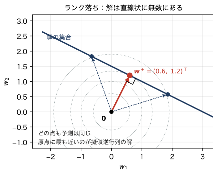
図 24 ランクが落ちた場合の解。直線上のどの点も同じ予測を与え、経験損失も等しい。擬似逆行列が選ぶのは、このうち原点に最も近い点（最小ノルム解）である。
