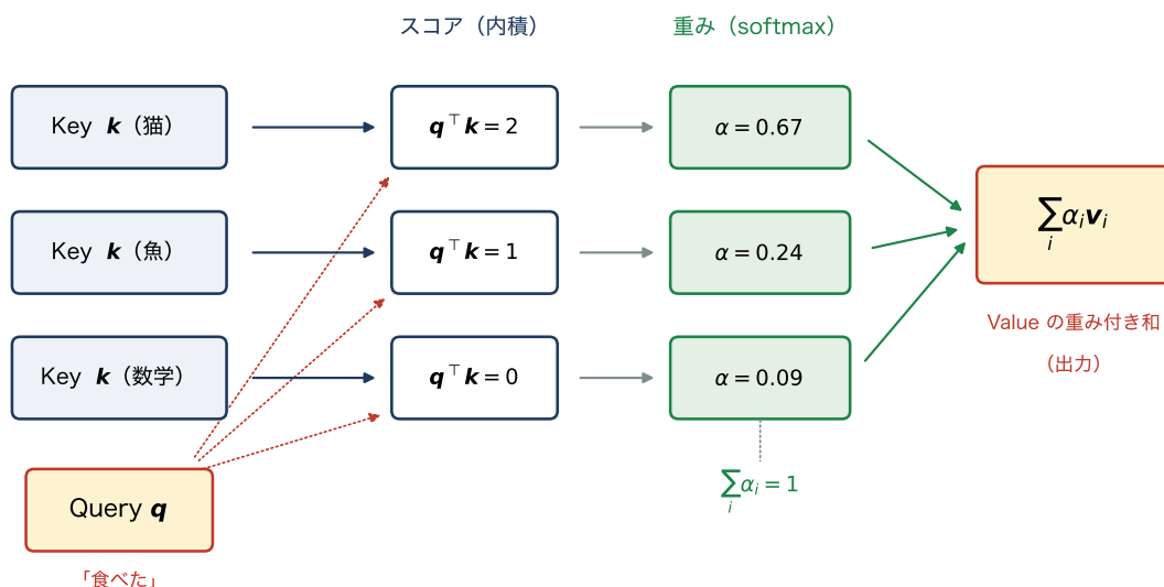
図 2.5 Attention のデータフロー。Query と各 Key の内積でスコアを計算し、ソフトマックスで重みに変換して、Value を混ぜ合わせる。
