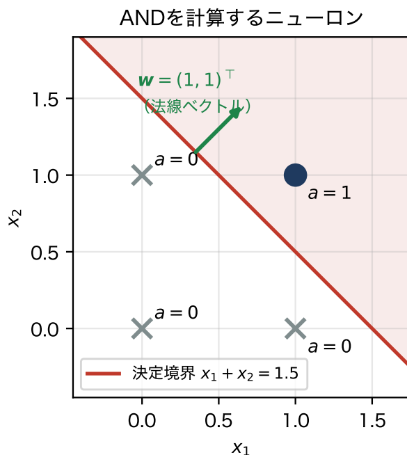
図 2.8 AND を計算するニューロン。決定境界 x_1 + x_2 = 1.5 が点 (1, 1) とそれ以外を分離し、重み \mathbf{w} は境界の法線ベクトルになっている。
