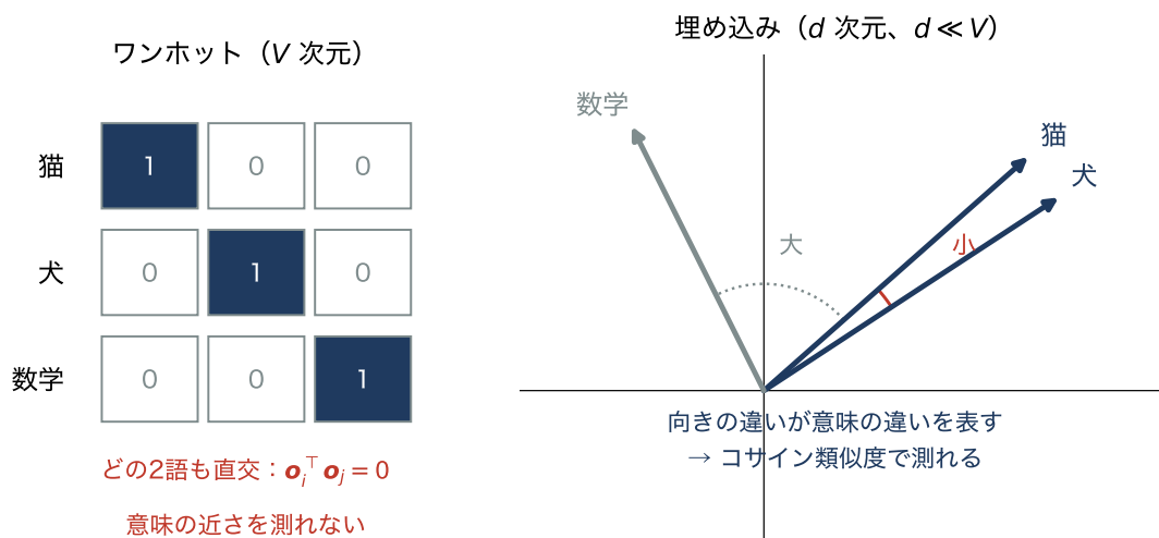
図 2.4 ワンホット表現と埋め込み。ワンホットではどの2語も直交するため意味の近さを測れないが、埋め込みでは向きの違いが意味の違いを表す。
