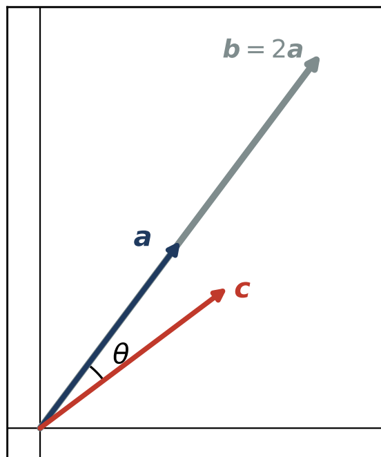
図 2.3 長さや向きの違い。 b = 2a は a より長いですが向きは同じなので \text{cossim}(a, b) = 1 である。
