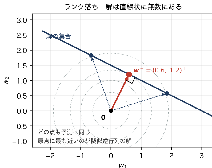
図 4.6 ランクが落ちた場合の解。直線上のどの点も同じ予測を与え、経験損失も等しい。擬似逆行列が選ぶのは、このうち原点に最も近い点（最小ノルム解）である。
