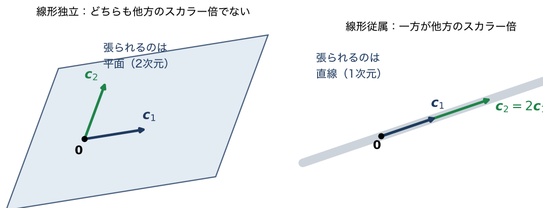
図 3.2 線形独立と線形従属 (模式図)。左：2 本が平行でなければ、線形結合は平面 (2 次元) を張る。右：一方が他方のスカラー倍であれば、どう線形結合しても直線 (1 次元) から出られない。
