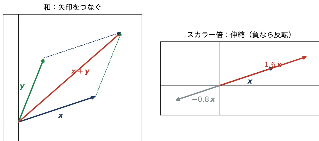
図 2.1 ベクトルの和とスカラー倍の幾何学的な意味。
