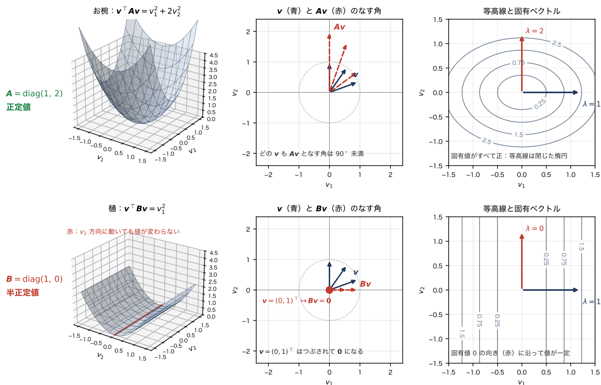
図 4.5 正定値（上段： A = \text{diag}(1, 2) ）と半正定値（下段： B = \text{diag}(1, 0) ）の 3 つの見方。左：2 次形式 v^T A v のグラフはお椀、 v^T B v は v_2 方向に平らな樋になる。中： v （青）と Av （赤）のなす角はつねに 90^\circ 未満だが、 B は v = (0, 1)^T を 0 につぶす。右： A の等高線は閉じた楕円で固有値はすべて正、 B は固有値 0 の固有ベクトルの向きに沿って値が一定で、等高線が閉じない。
