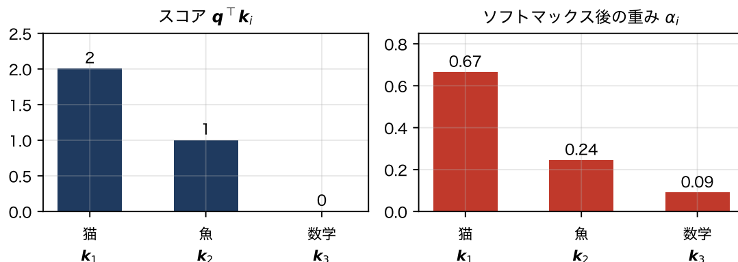
図 2.6 内積で計算したスコアと、ソフトマックスによる重み。スコアの差が指数関数で強調され、合計が 1 になる。
