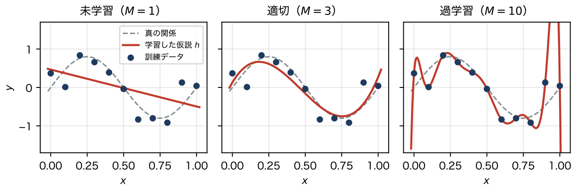
図 1.1 同じ訓練データに対する 3 つの仮説。仮説空間が小さすぎると構造を捉えられず (左)、大きすぎるとノイズまで再現してしまう (右)。
