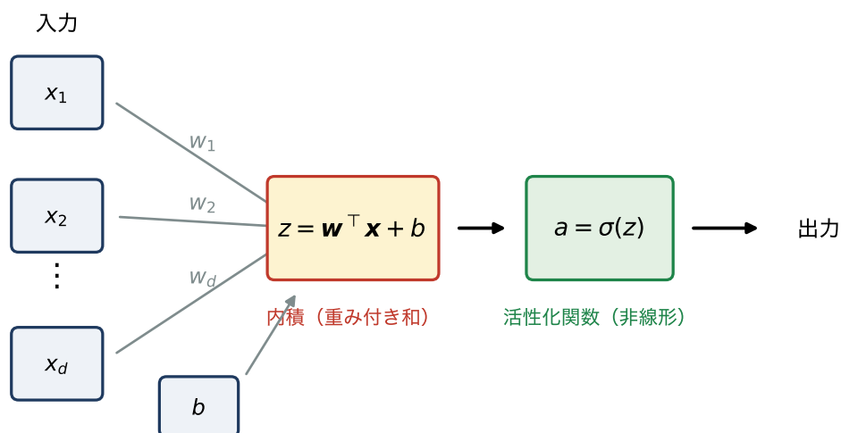
図 2.7 ニューロン 1 個の計算。入力と重みの内積にバイアスを加え（線形部分）、活性化関数を通す（非線形部分）。
