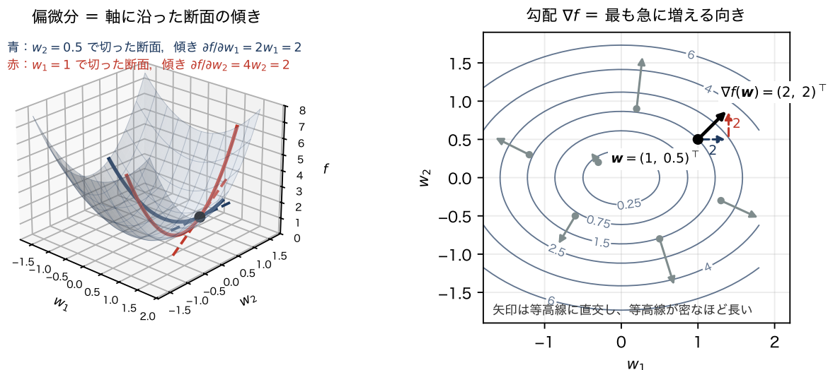
図 4.3 f(w_1, w_2) = w_1^2 + 2w_2^2 における偏微分と勾配。左：偏微分は曲面を各軸に平行に切った断面（青・赤の曲線）の傾き（破線）である。右：同じ関数の等高線と勾配ベクトル。点 (1, 0.5)^T での勾配 (2, 2)^T は 2 つの偏微分を成分に持ち、灰色の矢印も含めすべて等高線に直交する。
