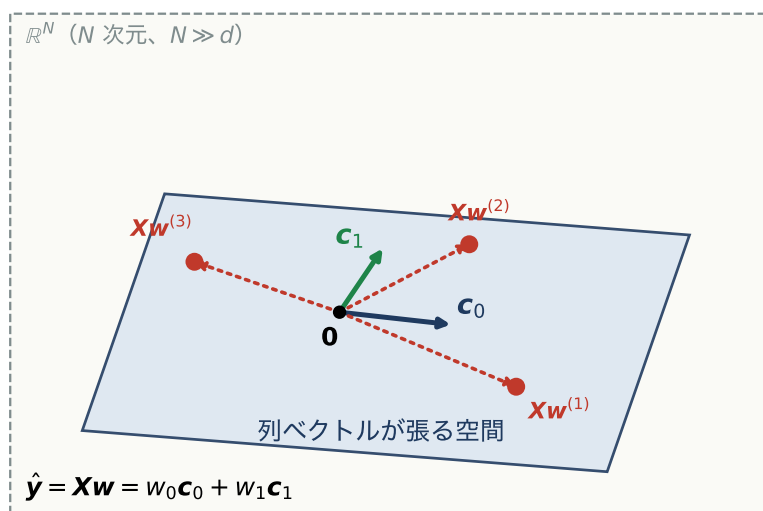
図 3.5 w を動かしたときの予測 \hat{y} = Xw の動く範囲。 w をどう選んでも \hat{y} は列ベクトルの張る部分空間から出られない。図は \text{rank}(X) = 2 の場合（平面）を描いた模式図である。
