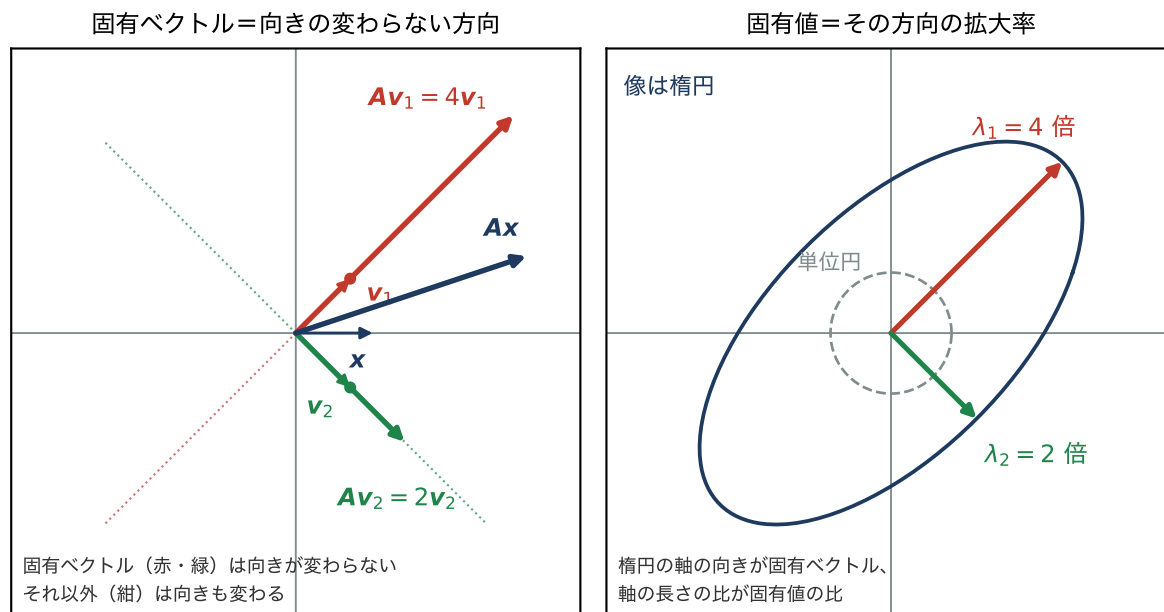
図 3.8 A = \begin{pmatrix} 3 & 1 \\ 1 & 3 \end{pmatrix} による変換。左: 固有ベクトル v_1, v_2 は向きが変わらず、長さだけがそれぞれ 4 倍、2 倍になる。固有ベクトルでない x は向きまで変わる。右: 単位円の像は楕円になり、楕円の軸の向きが固有ベクトル、軸の長さの比が固有値に対応する。
