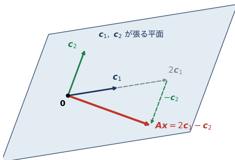
図 3.1 見方 2（列の線形結合）の幾何学的な意味（模式図）。 \mathbf{Ax} は列ベクトル \mathbf{c}_1, \mathbf{c}_2 の線形結合であるから、 \mathbf{x} をどう選んでも、2 本の列が張る平面の上にしか現れない。
