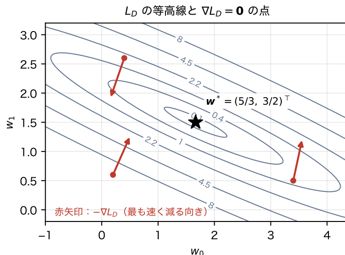
図 4.4 後述の数値例 ( D = \{(1, 3), (2, 5), (3, 6)\} ) における経験損失の等高線。赤い矢印は -\nabla L_D 、すなわち損失が最も速く減る向きである。中央の \mathbf{w}^* では勾配が \mathbf{0} になり、どの向きに動いても損失は増える。
