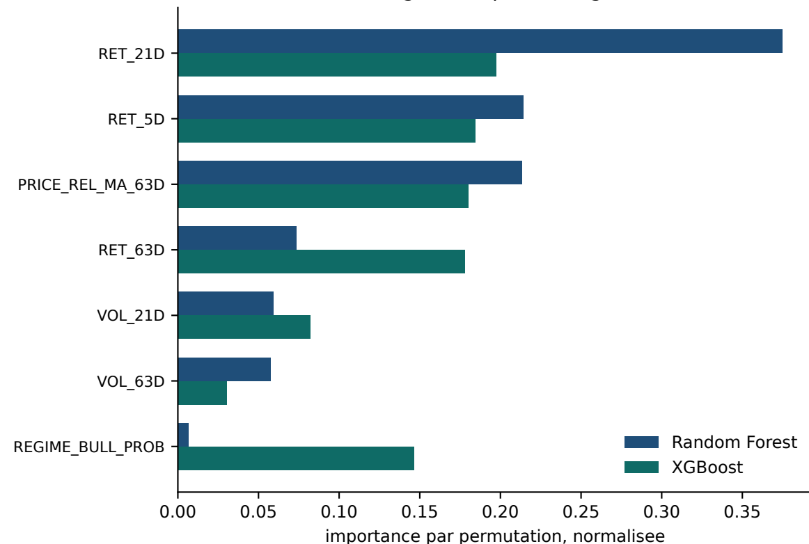
Challengers : importance globale
