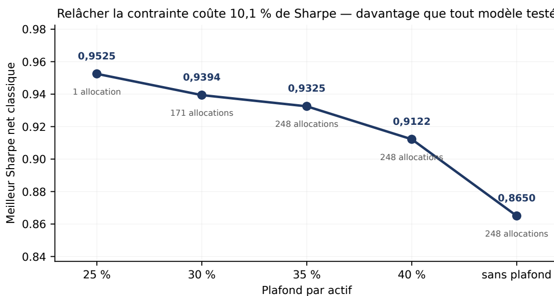
FIG. 5.5: Meilleur ratio de Sharpe classique en fonction du plafond par actif, sur 248 rééquilibrages et 20,7 ans. Le nombre d'allocations distinctes émises est indiqué sous chaque point.
