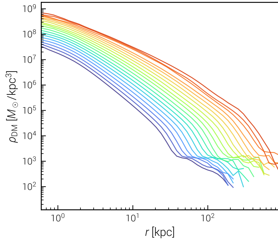
CDM-Dark
