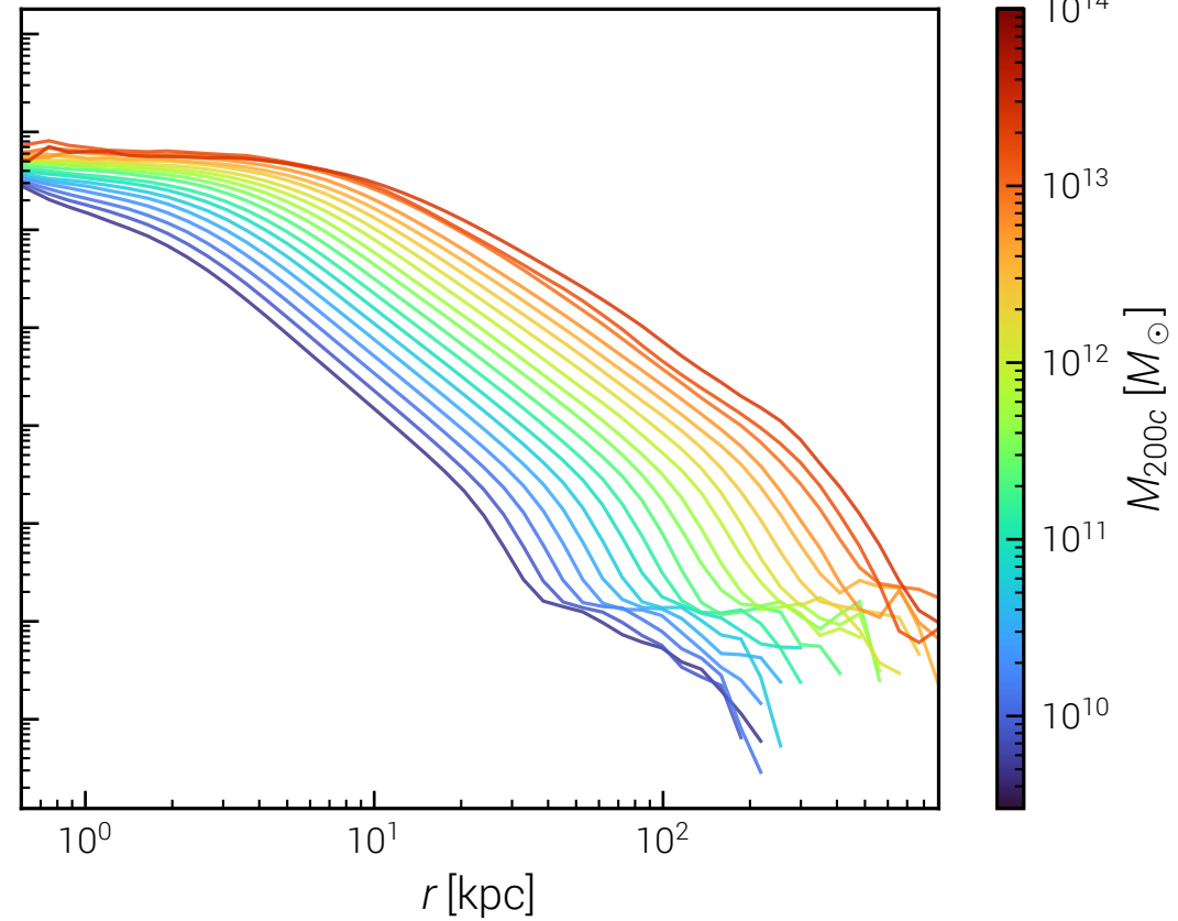
vSIDM-Dark (z=0.50)
