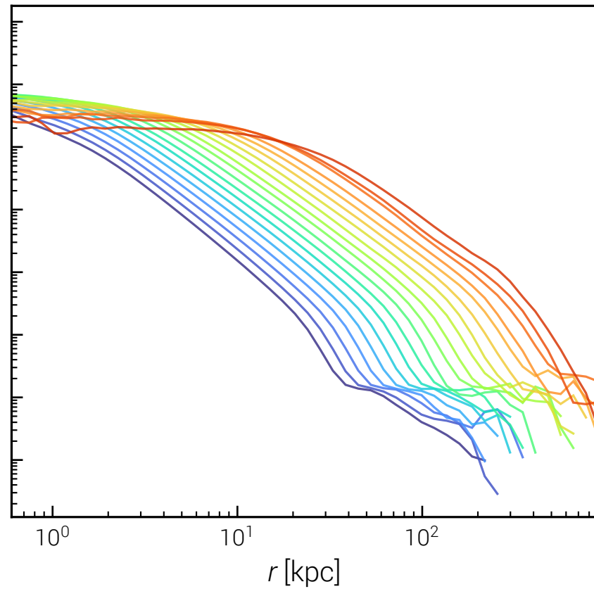
SIDM1-Dark
