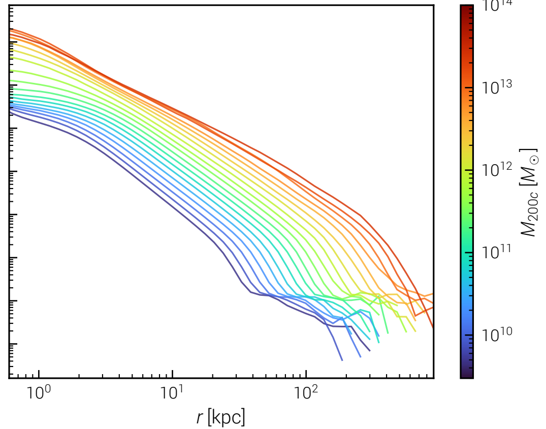
vSIDM ( z=0.50 )
