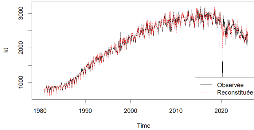
FIGURE 16 – Série observée vs série reconstituée \text{SARIMA}(2,1,4)(0,1,1)[12]
