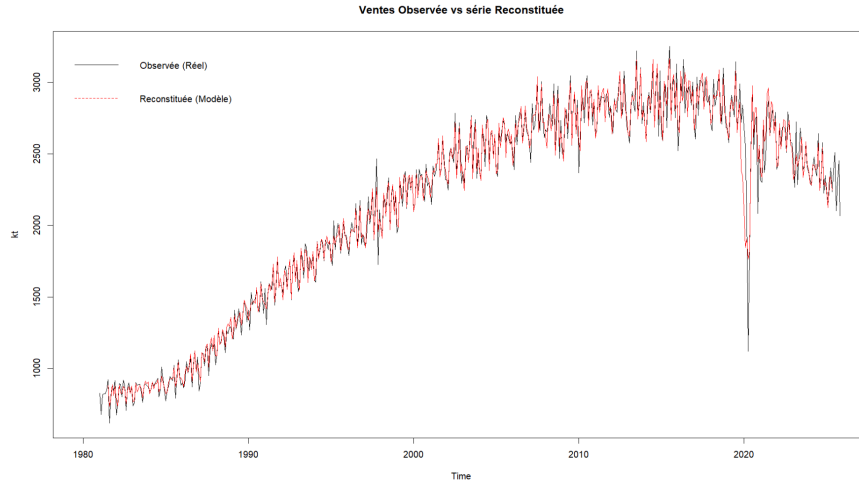
FIGURE 17 – Série observée vs série reconstituée \text{ARMA}(4,4)
