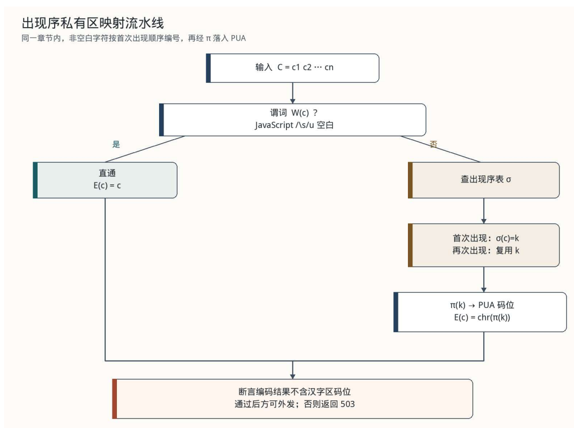
图 4-3 单字符编码流程
