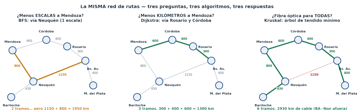
Figura 11.12: La misma red, tres preguntas. Izquierda: BFS minimiza tramos — a Mendoza por Neuquén, 1 escala, pero 1950 km. Centro: Dijkstra minimiza kilómetros — por Rosario y Córdoba, 3 tramos pero 1300 km. Derecha: Kruskal conecta las 7 ciudades con 2930 km de fibra, descartando la ruta más redundante (BA–Neuquén).
