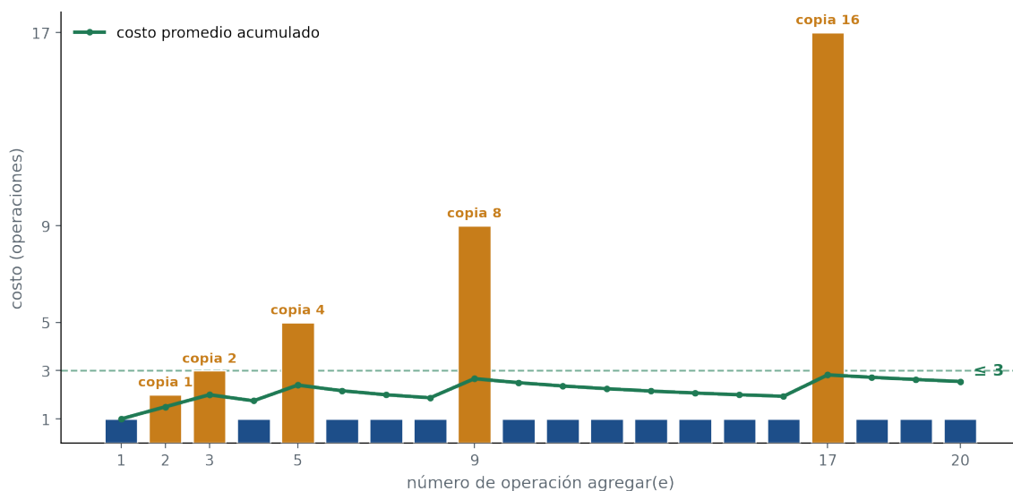
Figura 4.8: El costo de cada operación agregar con redimensión por duplicación. Casi todas cuestan 1 (azul); las que caen justo en una redimensión (naranja) pagan además la copia de todo lo existente. La línea verde —el promedio acumulado— nunca supera 3.
