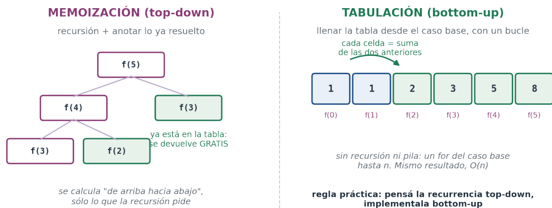
Figura 10.5: Memoización (top-down): la recursión natural más una tabla que evita recalcul — los subproblemas repetidos se devuelven gratis. Tabulación (bottom-up): un bucle llena la tabla desde el caso base. Regla práctica: pensá la recurrencia top-down, implementala bottom-up.
