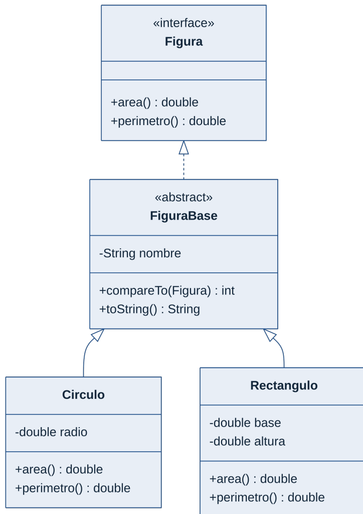
Figura 3.10: El TDA Figura (interfaz), la clase abstracta FiguraBase y las figuras concretas.
