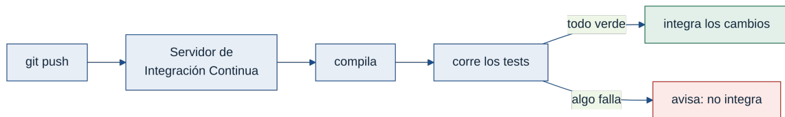
Figura 3.11: Integración continua: cada push dispara compilar y testear; si algo falla, avisa.
