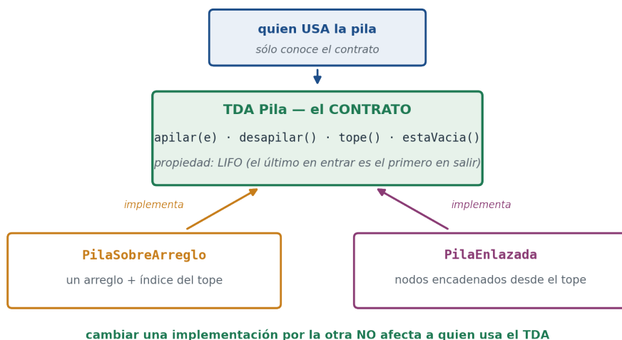
Figura 3.1: El TDA como contrato: quien usa la Pila conoce sólo sus operaciones y su propiedad LIFO. Abajo, dos implementaciones intercambiables: cambiar una por otra no afecta al usuario.
