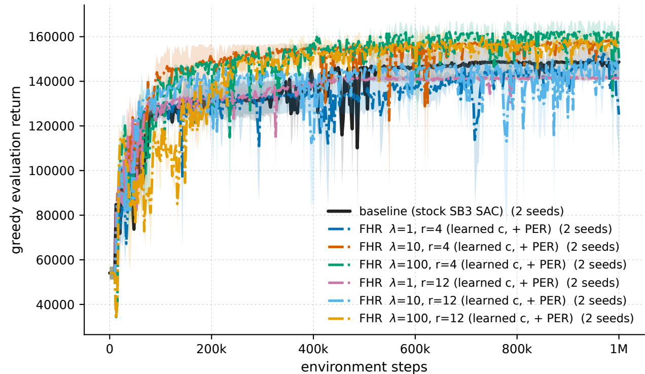
HumanoidStandup-v5 - all arms (eval)
