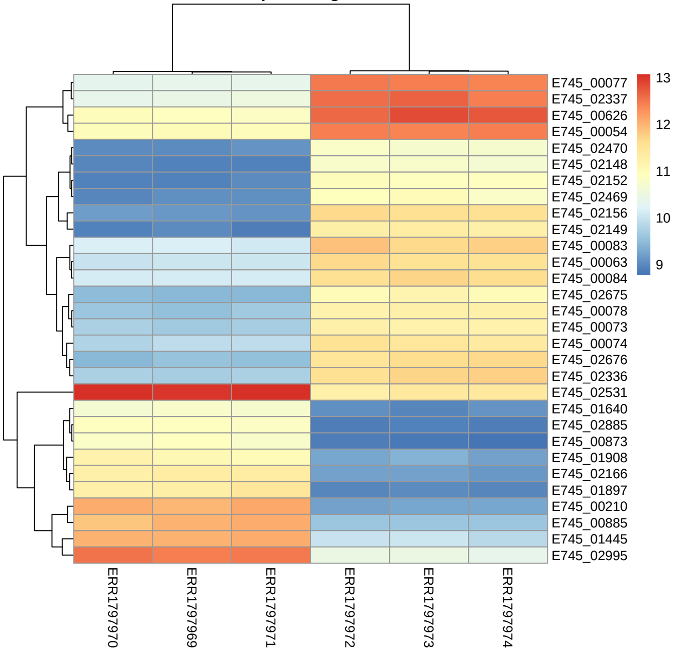
Top 30 DE genes
