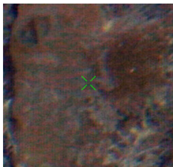
AA2011_CTD135
