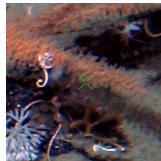
AA2011_CTD75
