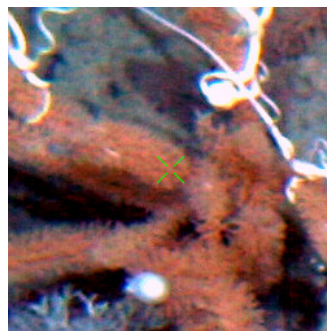
AA2011_CTD114
