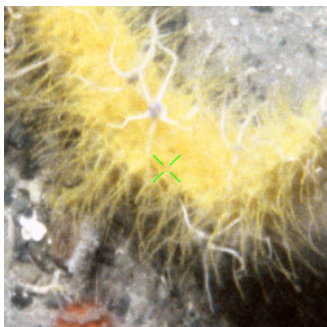
PS18_165
