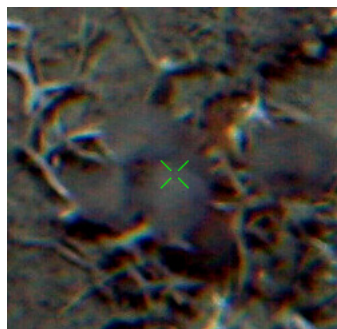
AA2011_CTD72
