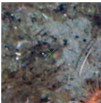
AA2011_CTD109
