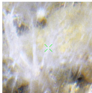
PS18_180
