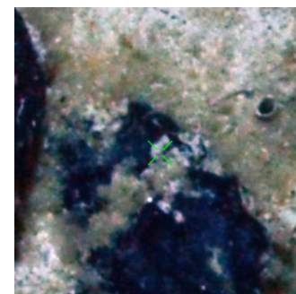
TAN1802_213
