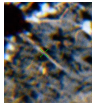
PS14_259
