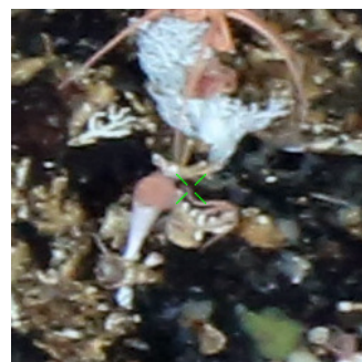
PS118_69
