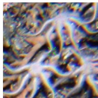
tan0802_150
