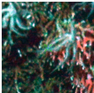
tan1901_164
