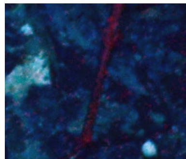
TAN1802_184
