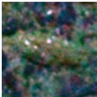
tan1901_183
