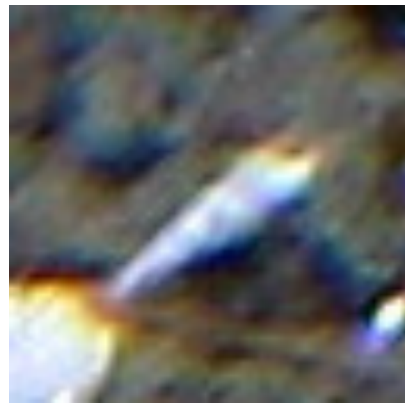
tan0802_108
