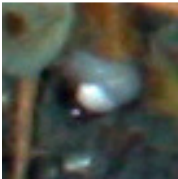
PS81_197
