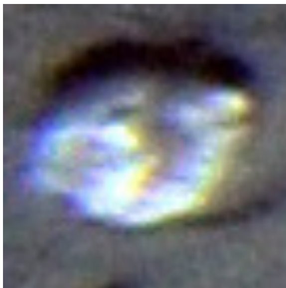
LMG1311_3
