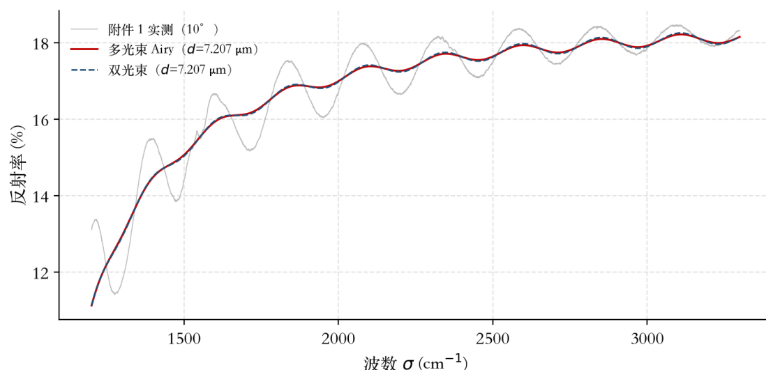
图 17: 碳化硅（附件 1）全谱复核：多光束 Airy 模型与双光束模型拟合结果几乎重合，多光束项未带来拟合优度改善。
