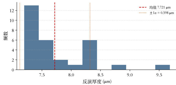
图 19: 蒙特卡洛噪声实验 (0.3% 反射率噪声, 30 次) 的反演厚度分布。
