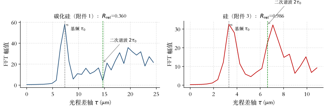
图 12: 多光束干涉的频域二次谐波判据：碳化硅（左）与硅（右）反射谱在光程差轴上的 FFT 幅值谱。硅的谐波相对强度 R_{\text{rel}} = 0.986 ，显著高于碳化硅的 0.360。
