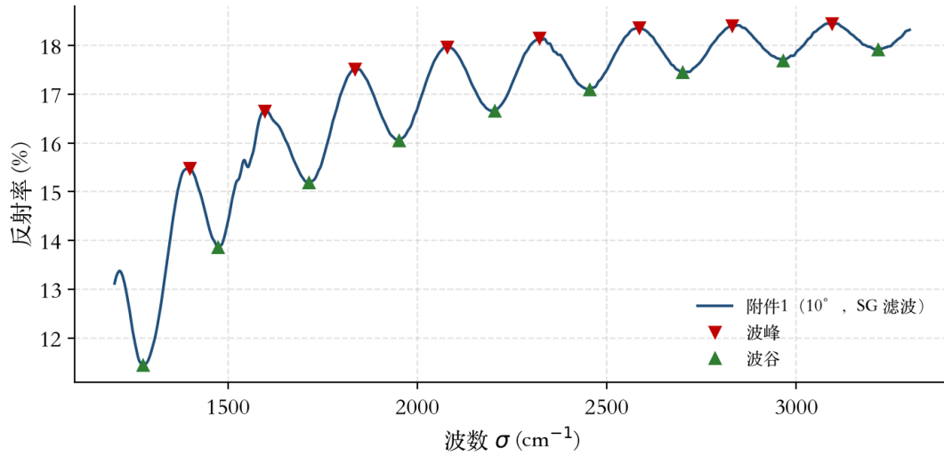
图 6: 附件 1 ( 10^\circ ) SG 滤波谱上的极值检测结果 ( \sigma \in [1200, 3300]\ \text{cm}^{-1} )。
