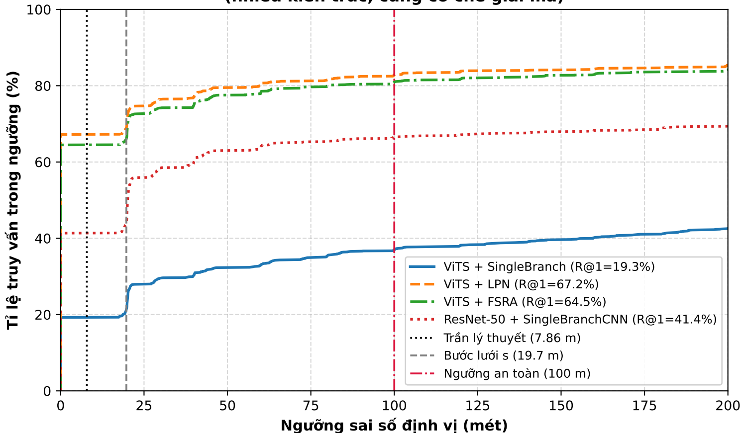
Hình 1: Phân bố tích lũy sai số định vị (CDF) (nhiều kiến trúc, cùng cơ chế giải mã)
