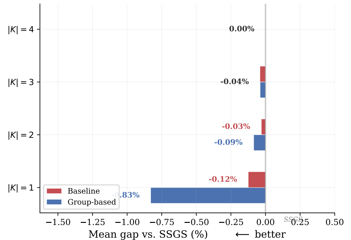
(d) Improvement over SSGS warm-start
