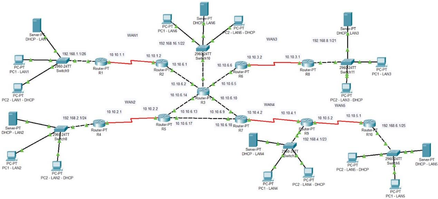
Figura 2: Rede com a adição de PCs e DHCP.
