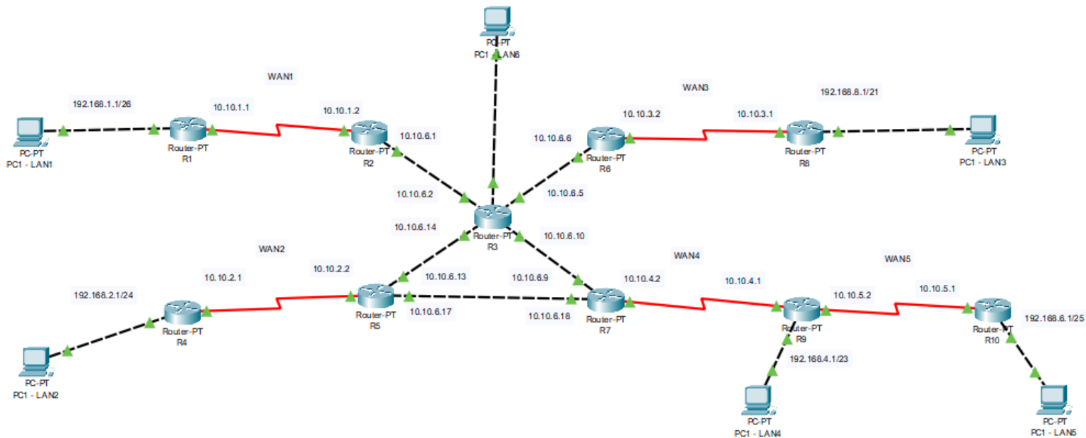
Figura 1: Rede utilizada para o endereçamento de IP.
