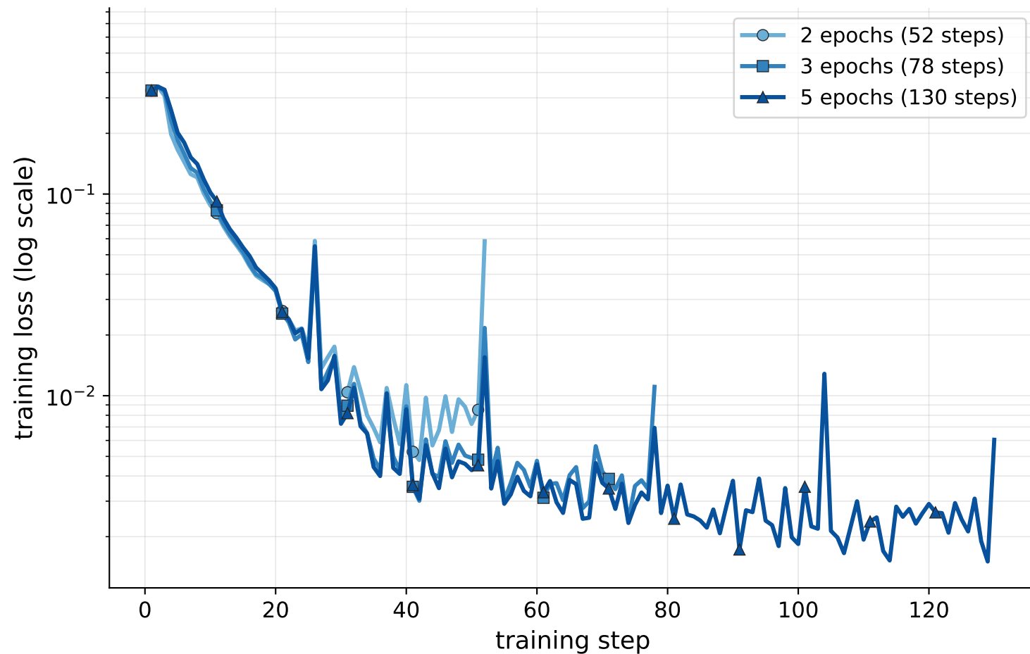
Gemma 4 E2B
