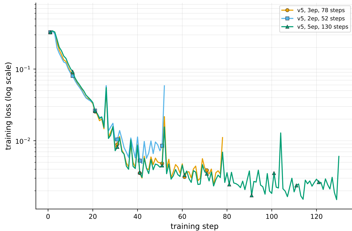
Gemma 4 E2B
