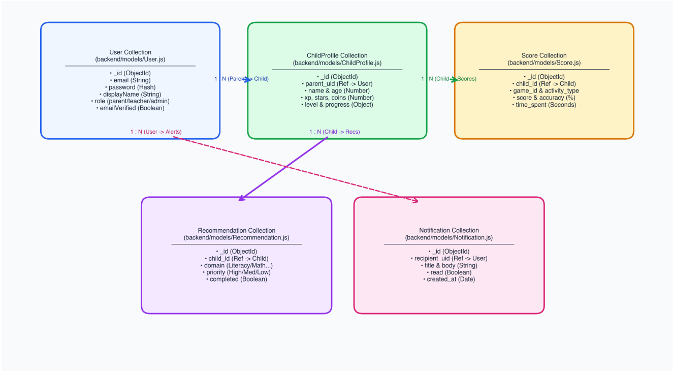
MongoDB Database Entity-Relationship & Schema Diagram (ERD)
