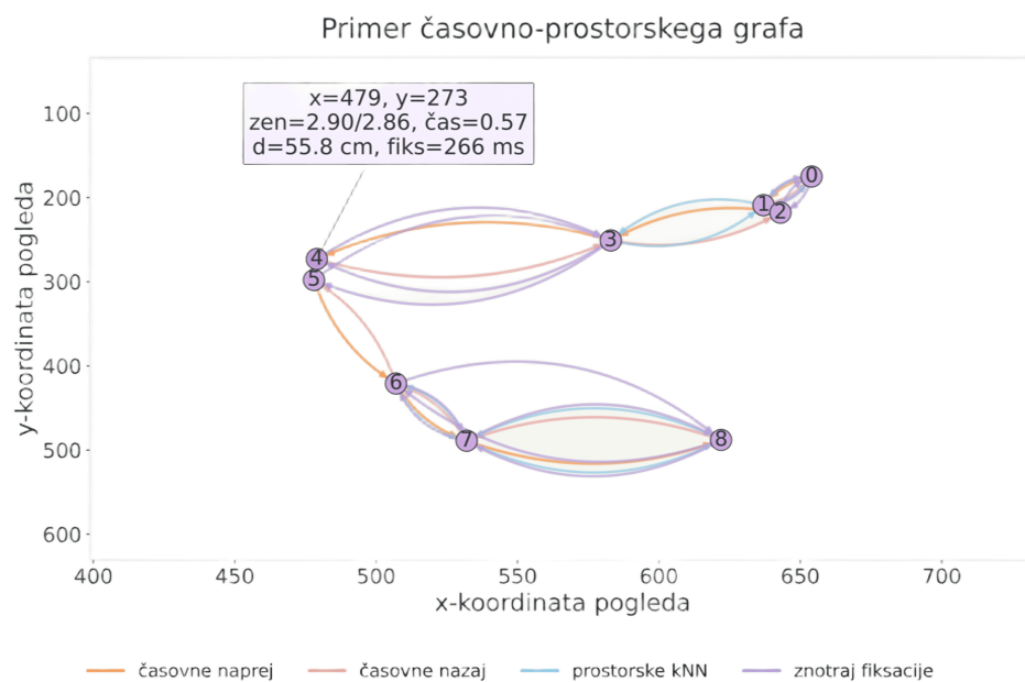
Slika 4.2: Primer grafovske konstrukcije za množico vsí signali . Vozlišča predstavljajo meritve v izseku časovnega okna, povezave pa prikazujejo časovne, prostorske in fiksacijske relacije. Ločeni prikazi posameznih relacij so zbrani v dodatku B.
