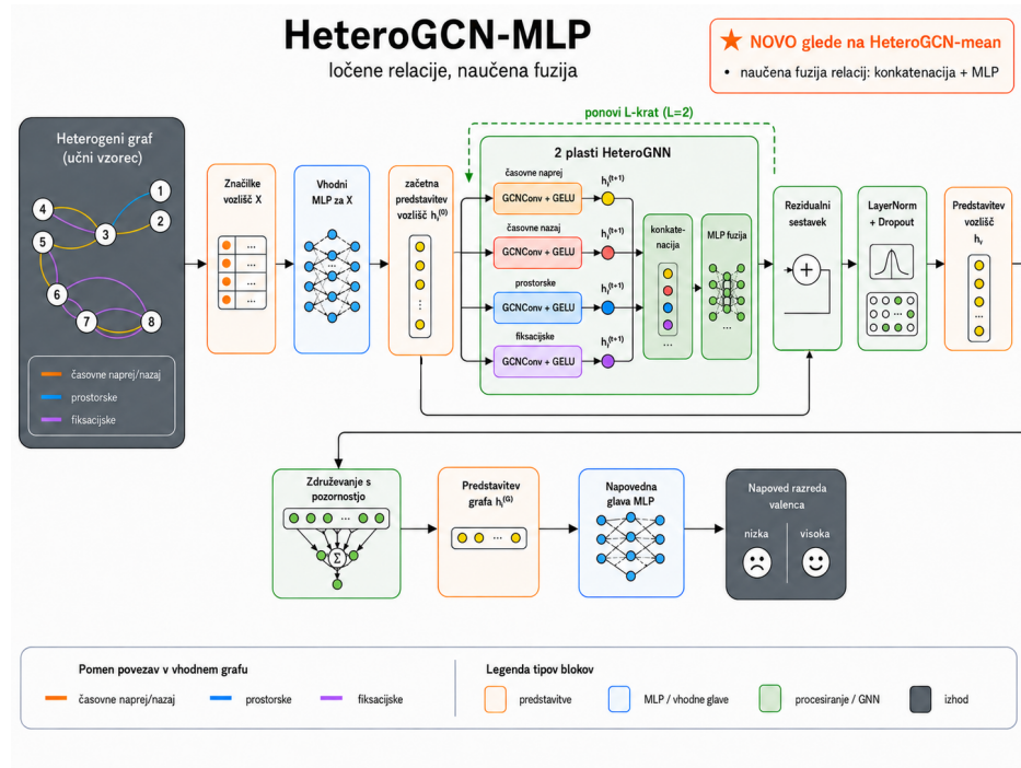
Slika 5.3: Diagram arhitekture HeteroGCN-MLP. Model relacijske predstavitve najprej konkatenera, nato pa jih združi z učljivo fuzijo prek dvoslojnega perceptrona.
