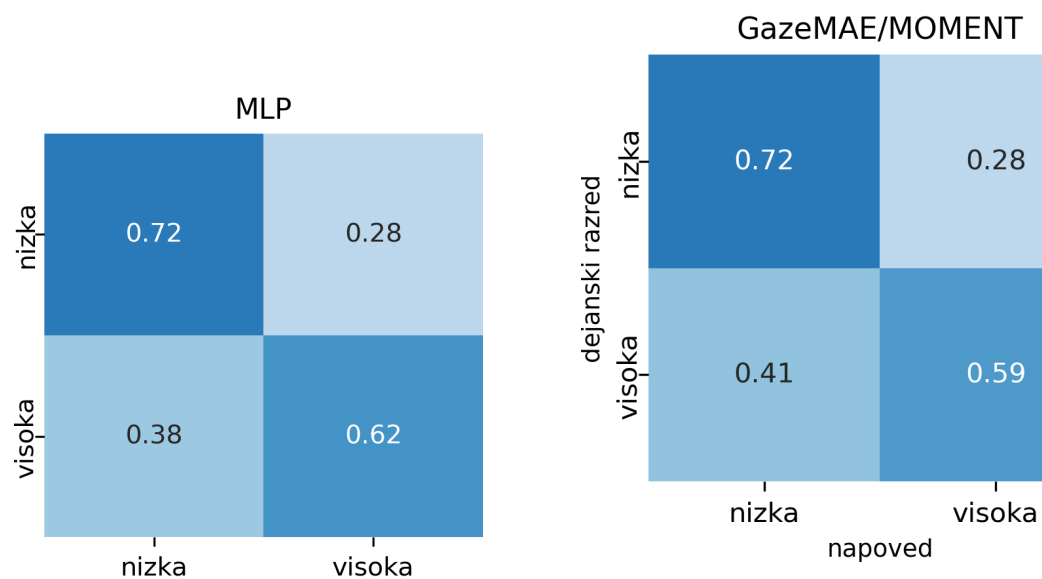
Slika A.3: Matriki zmede za množico signalov samo pogled: MLP in GazeMAE/MOMENT.
