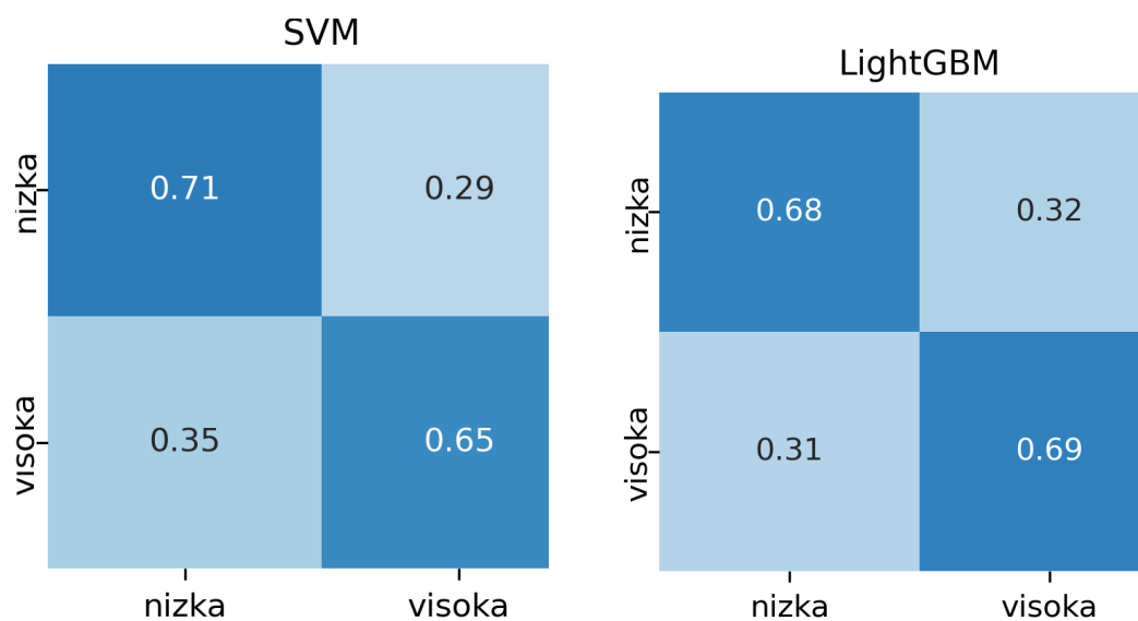
Slika A.17: Matriki zmede za množico signalov vsi signali: SVM in LightGBM.
