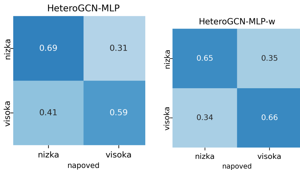
Slika A.15: Matriki zmede za množico signalov pogled in zenici: HeteroGCN-MLP in HeteroGCN-MLP-w.
