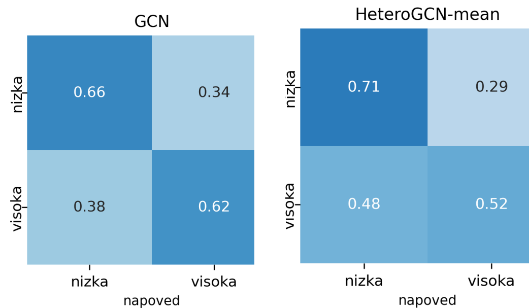
Slika A.4: Matriki zmede za množico signalov samo pogled: GCN in HeteroGCN-mean.
