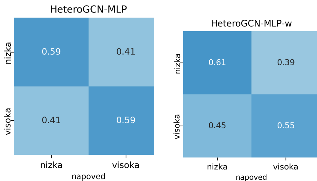
Slika A.10: Matriki zmede za množico signalov samo zenici: HeteroGCN-MLP in HeteroGCN-MLP-w.
