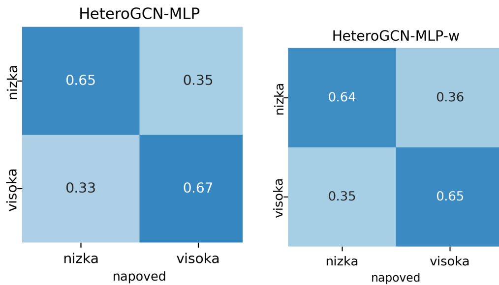
Slika A.5: Matriki zmede za množico signalov samo pogled: HeteroGCN-MLP in HeteroGCN-MLP-w.
