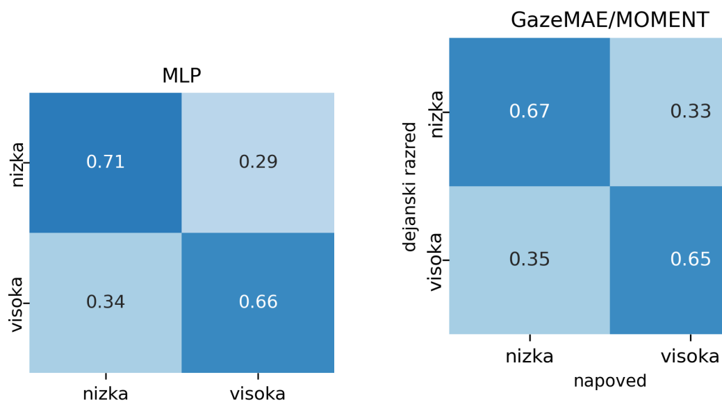
Slika A.13: Matriki zmede za množico signalov pogled in zenici: MLP in GazeMAE/MOMENT.
