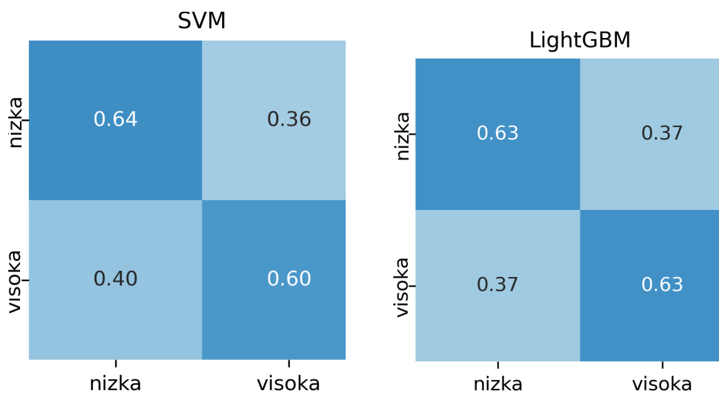
Slika A.7: Matriki zmede za množico signalov samo zenici: SVM in LightGBM.
