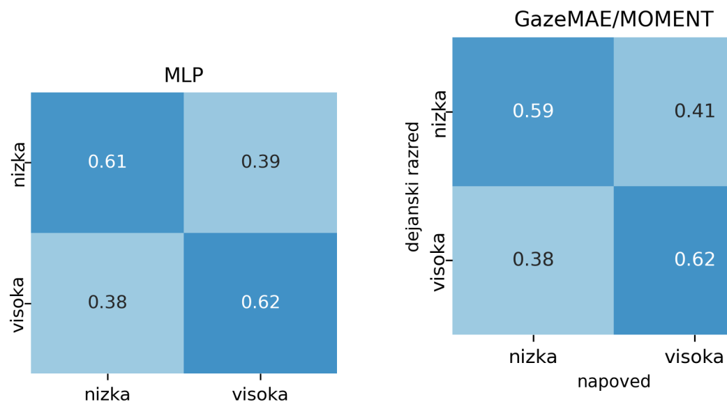
Slika A.8: Matriki zmede za množico signalov samo zenici: MLP in GazeMAE/MOMENT.
