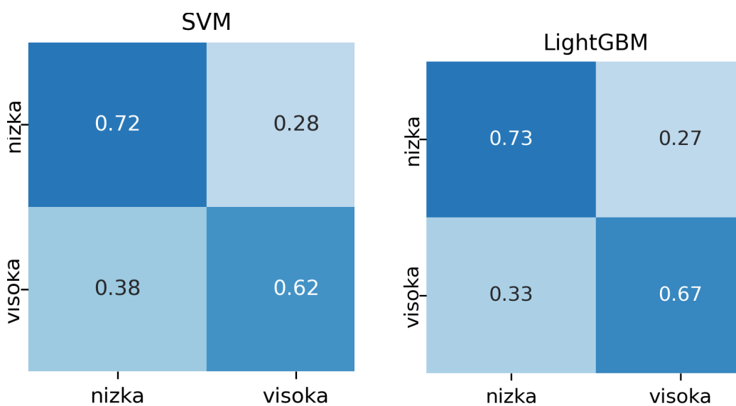
Slika A.2: Matriki zmede za množico signalov samo pogled: SVM in LightGBM.
