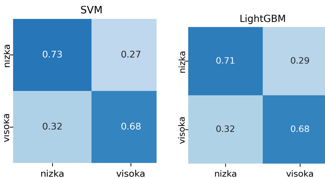
Slika A.12: Matriki zmede za množico signalov pogled in zenici: SVM in LightGBM.
