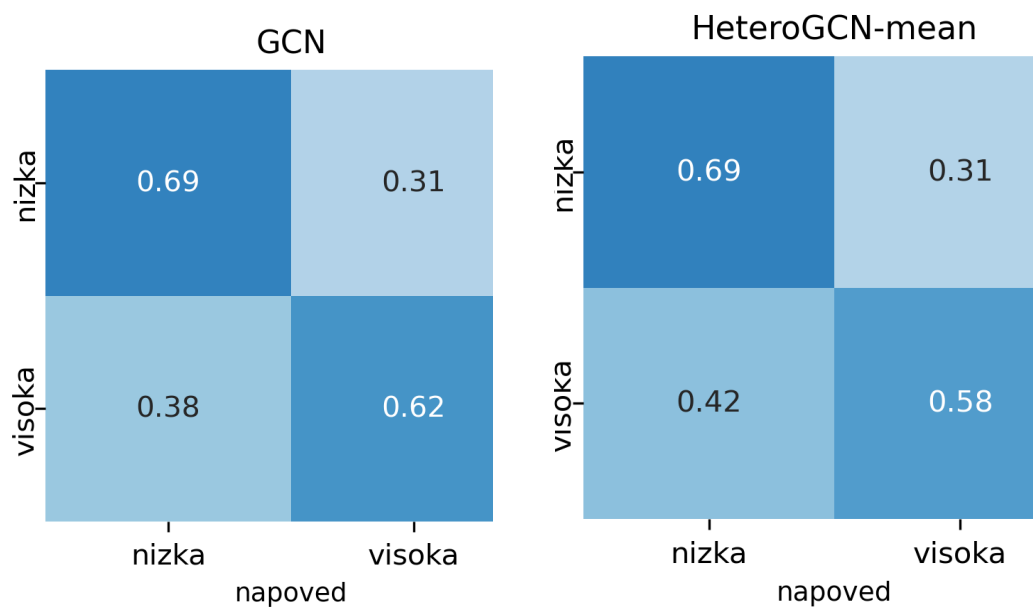
Slika A.14: Matriki zmede za množico signalov pogled in zenici: GCN in HeteroGCN-mean.
