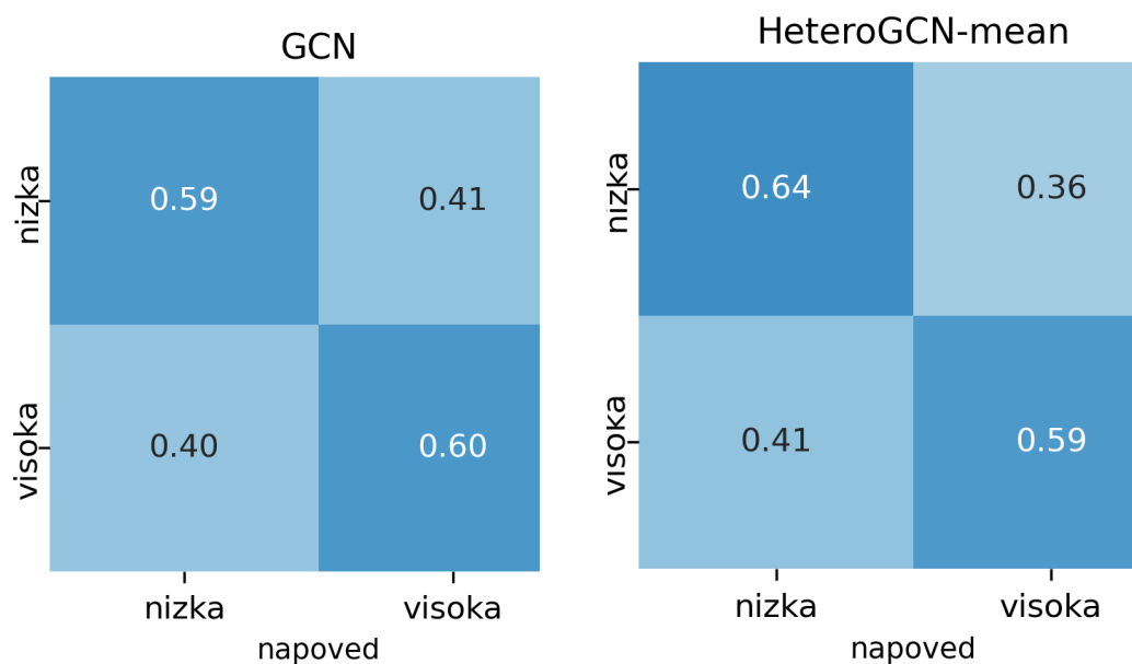
Slika A.19: Matriki zmede za množico signalov vsi signali: GCN in HeteroGCN-mean.
