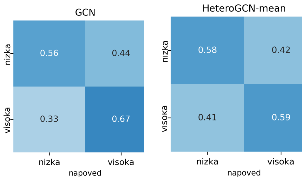
Slika A.9: Matriki zmede za množico signalov samo zenici: GCN in HeteroGCN-mean.
