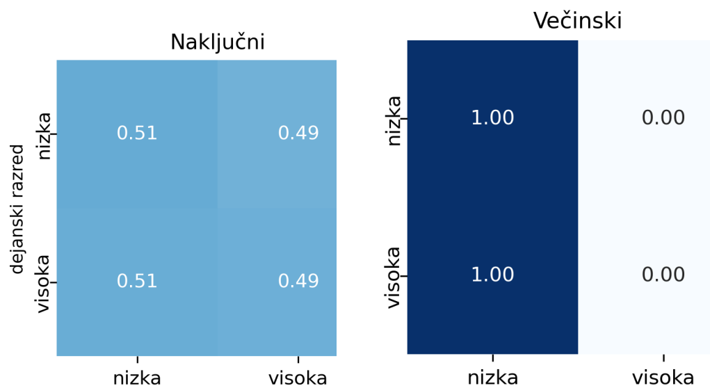
Slika A.1: Matriki zmede za množico signalov samo pogled: naključni in večinski model.
