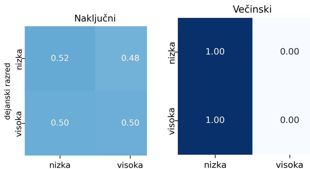
Slika A.6: Matriki zmede za množico signalov samo zenici: naključni in večinski model.
