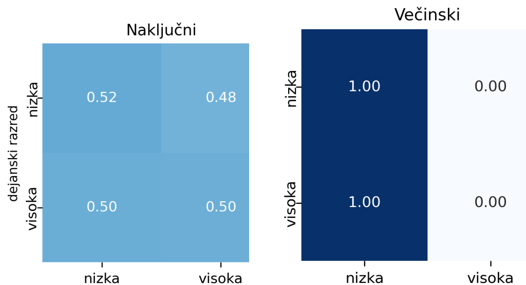
Slika A.11: Matriki zmede za množico signalov pogled in zenici: naključni in večinski model.
