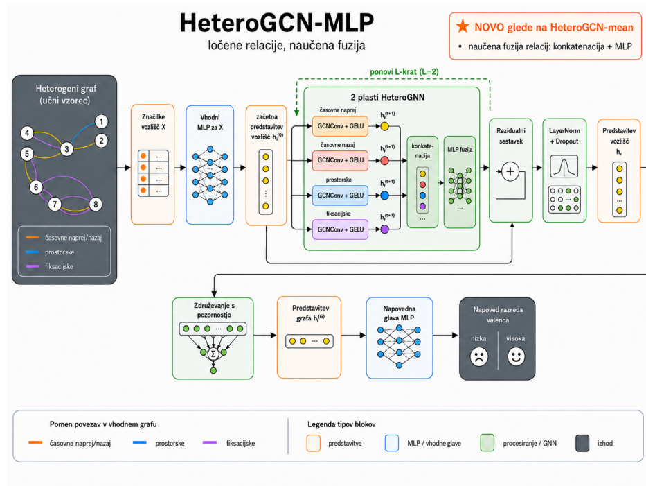
Slika 5.3: Diagram arhitekture HeteroGCN-MLP . Model relacijske predstavitve najprej konkatenuira, nato pa jih združi z učljivo fuzijo prek dvoslojnega perceptrona.
